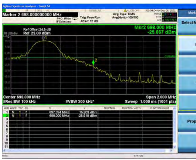
Band71 / 10MHz / High CH / QPSK / 1 RB
