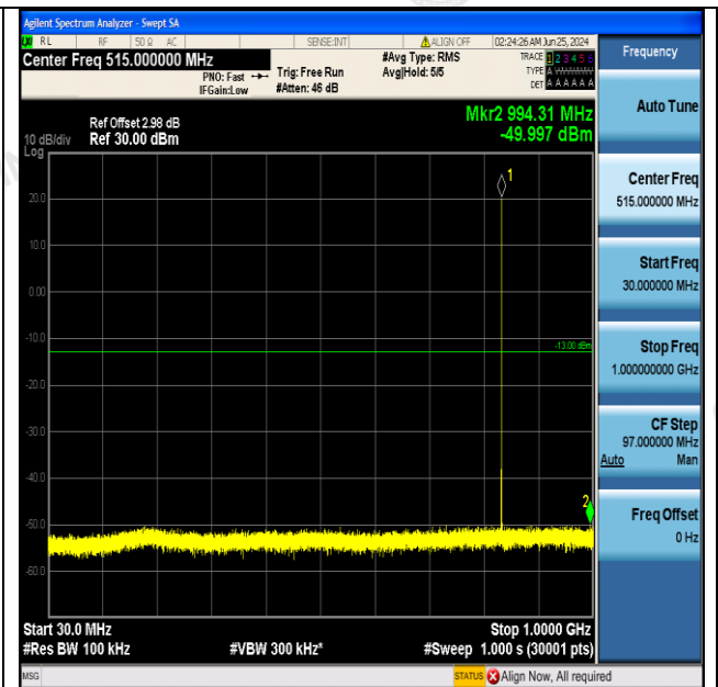
GPRS850-190-5-30~1000MHz-PASS
