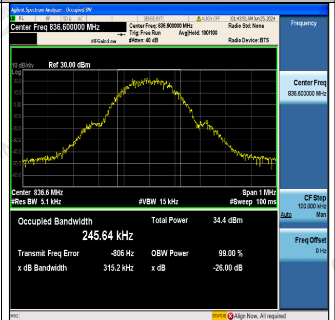
GPRS850-190-5-PASS
