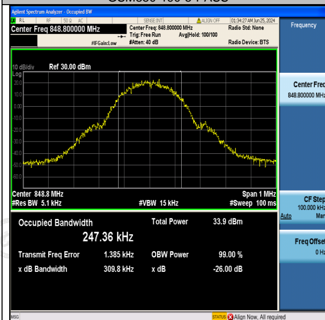
GSM850-251-5-PASS
