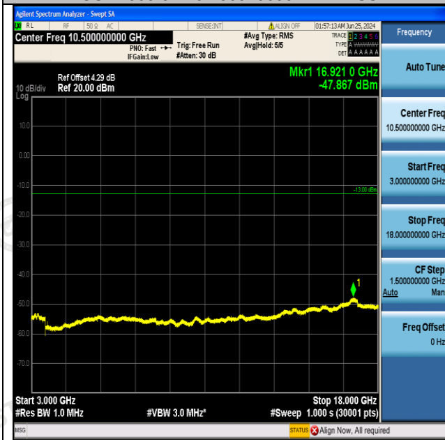
GSM1900-512-0-3000~18000MHz-PASS
