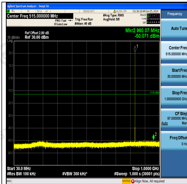
GSM850-190-5-30~1000MHz-PASS
