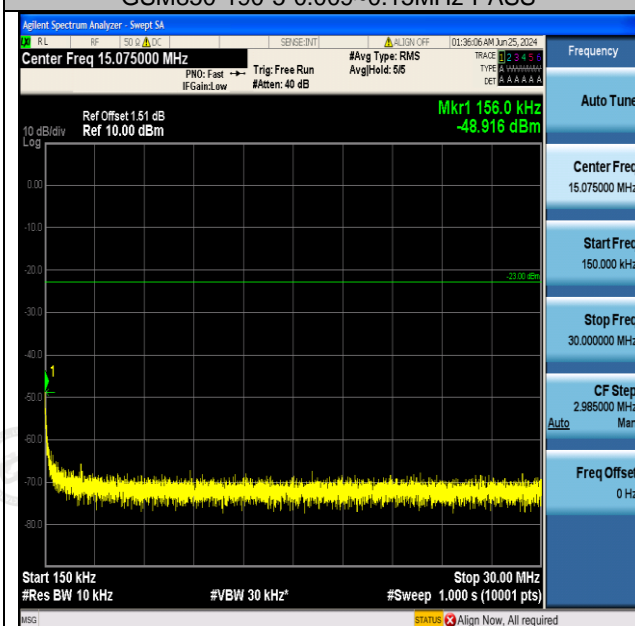
GSM850-190-5-0.15~30MHz-PASS
