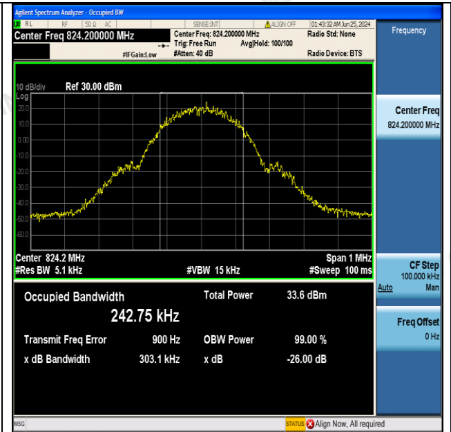
GPRS850-128-5-PASS
