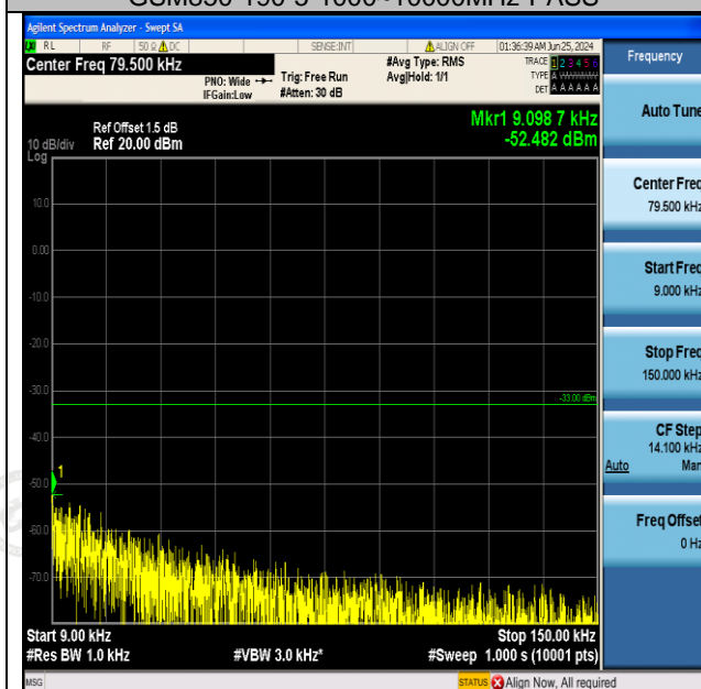
GSM850-251-5-0.009~0.15MHz-PASS
