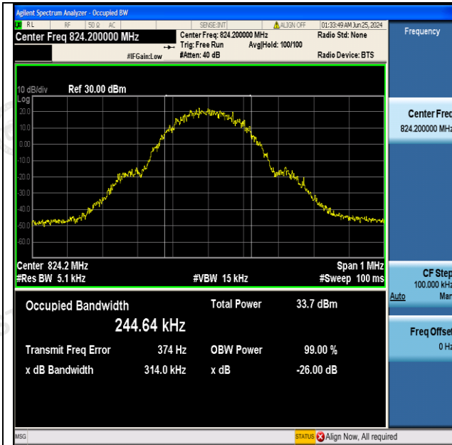
GSM850-128-5-PASS
