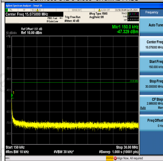
GSM1900-512-0-0.15~30MHz-PASS
