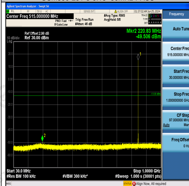
GSM850-251-5-30~1000MHz-PASS
