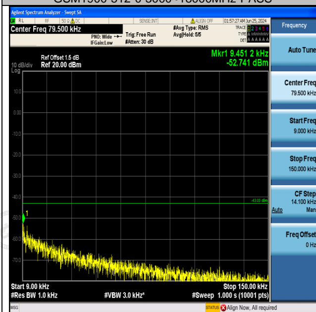
GSM1900-661-0-0.009~0.15MHz-PASS
