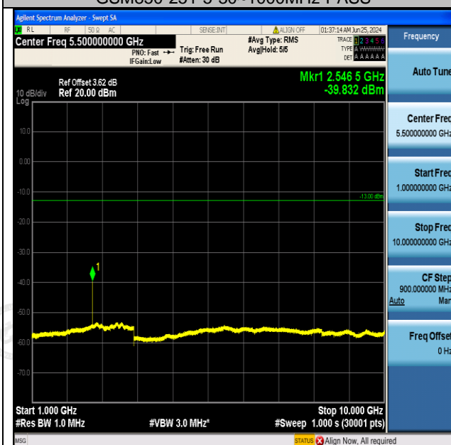
GSM850-251-5-1000~10000MHz-PASS
