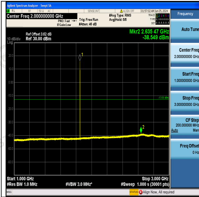
GSM1900-512-0-1000~3000MHz-PASS
