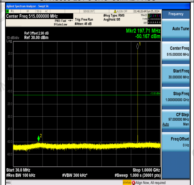
GPRS850-251-5-30~1000MHz-PASS
