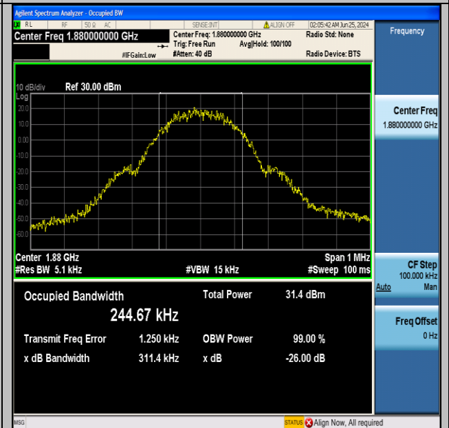
GPRS1900-661-0-PASS
