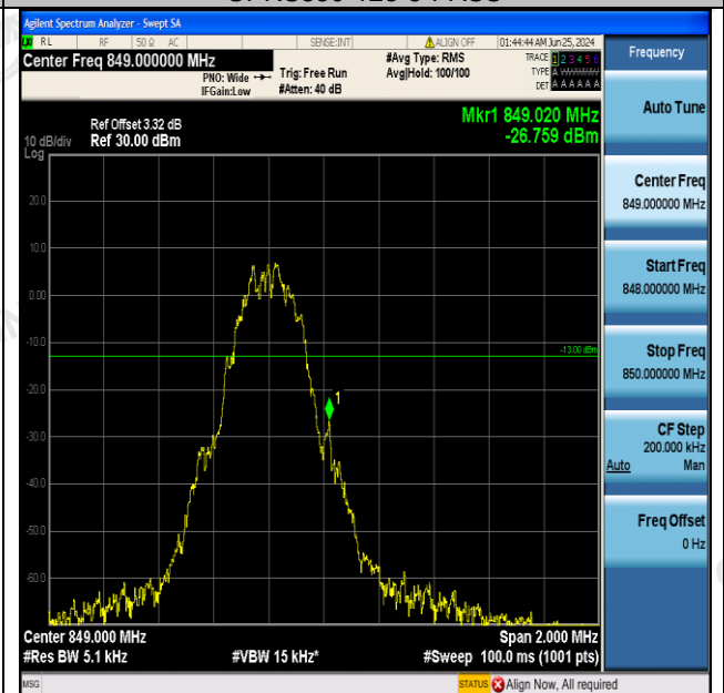
GPRS850-251-5-PASS
