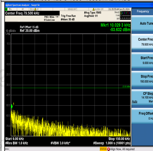
GSM850-190-5-0.009~0.15MHz-PASS
