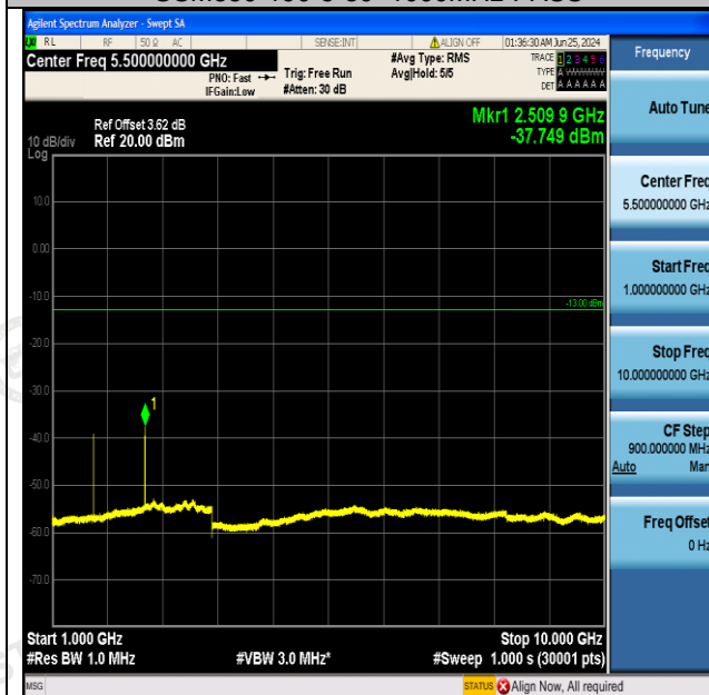
GSM850-190-5-1000~10000MHz-PASS
