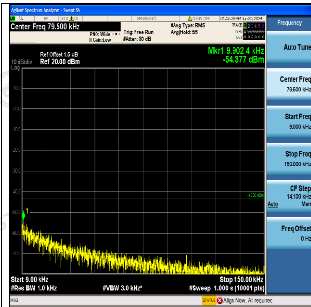
GSM1900-512-0-0.009~0.15MHz-PASS
