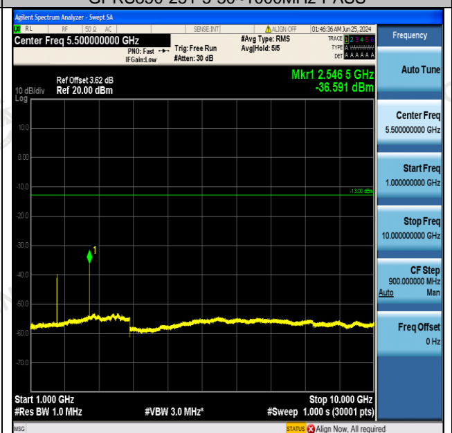
GPRS850-251-5-1000~10000MHz-PASS
