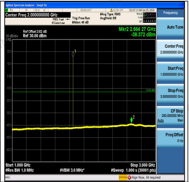
GPRS1900-512-0-1000~3000MHz-PASS
