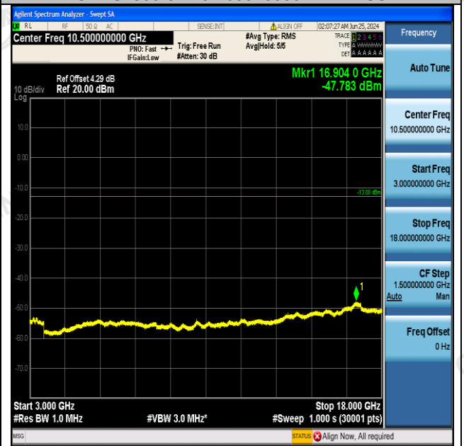
GPRS1900-512-0-3000~18000MHz-PASS
