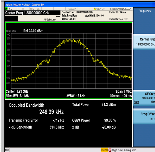
GSM1900-661-0-PASS
