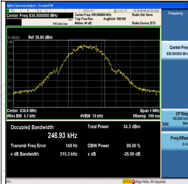
GSM850-190-5-PASS
