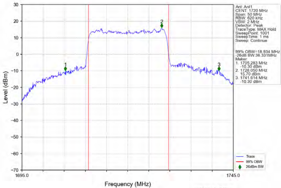
n66 30kHz SISO NTVN 20MHz CP-OFDM QPSK 1720MHz Outer Full
