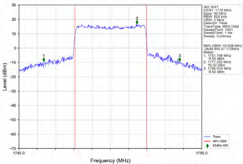
n66 15kHz SISO NTN 20MHz CP-OFDM QPSK 1770MHz Outer Full
