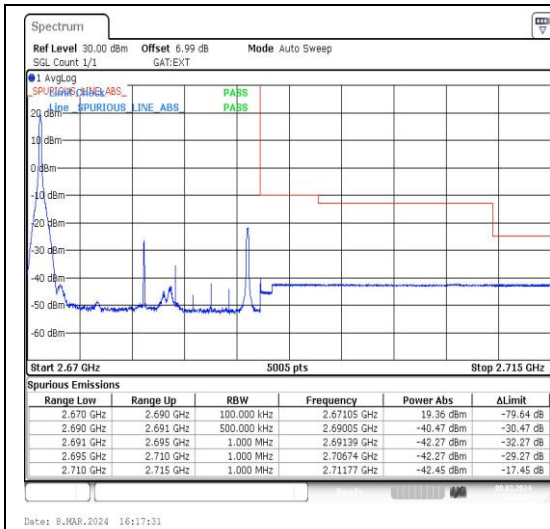
Band41_20MHz_QPSK_41490_1RB#0
