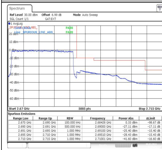
Band41_20MHz_QPSK_41490_1RB#99
