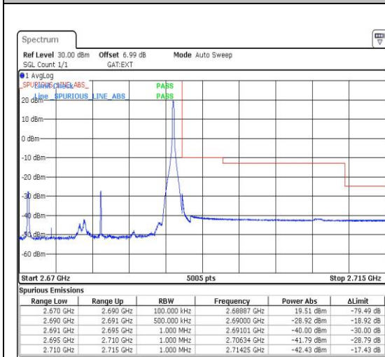
Band41_20MHz_QPSK_41490_1RB#0
