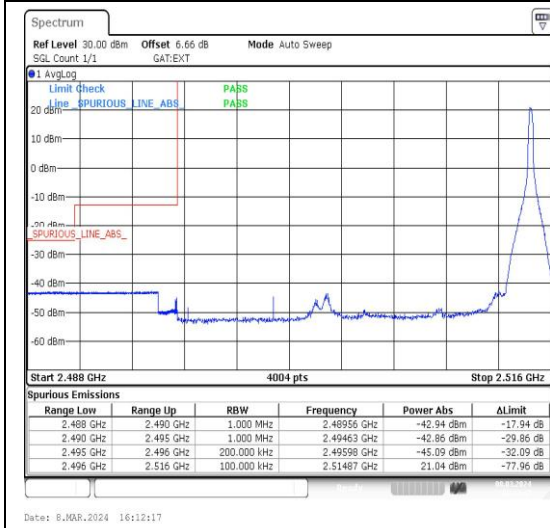
Band41_20MHz_QPSK_39750_1RB#99
