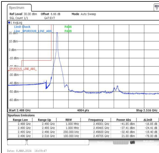
Band41_20MHz_QPSK_39750_1RB#0
