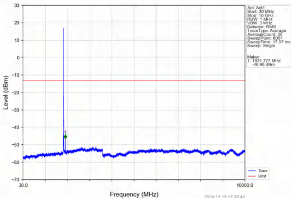
Band2 10MHz QPSK LCH 1855MHz RB 1 0 NTV
