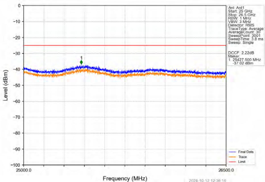
Band41_20MHz_QPSK_MCH_2593MHz_RB_1_0 NTN
