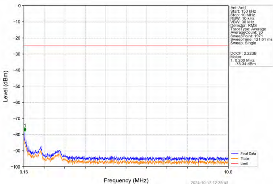
Band41_20MHz_QPSK_MCH_2593MHz_RB_1_0_NTNV
