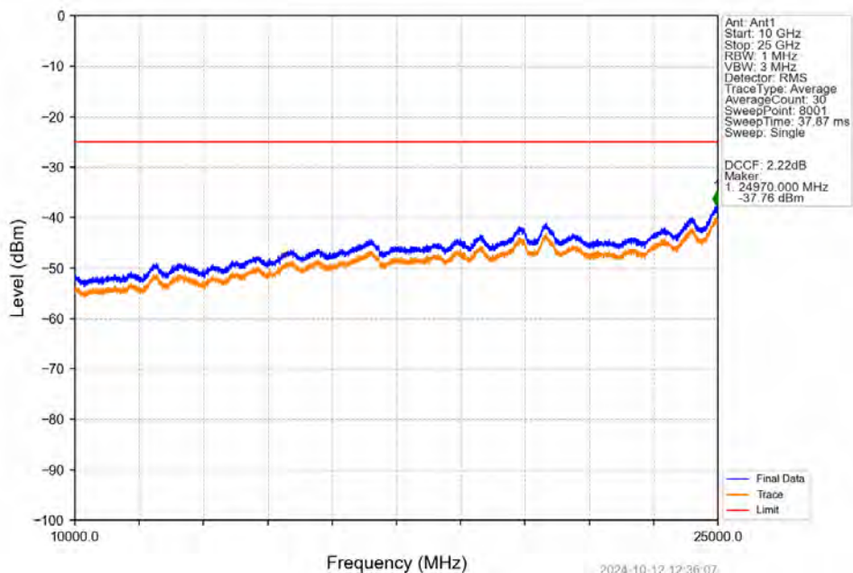
Band41_20MHz_QPSK_MCH_2593MHz_RB_1_0 NTN
