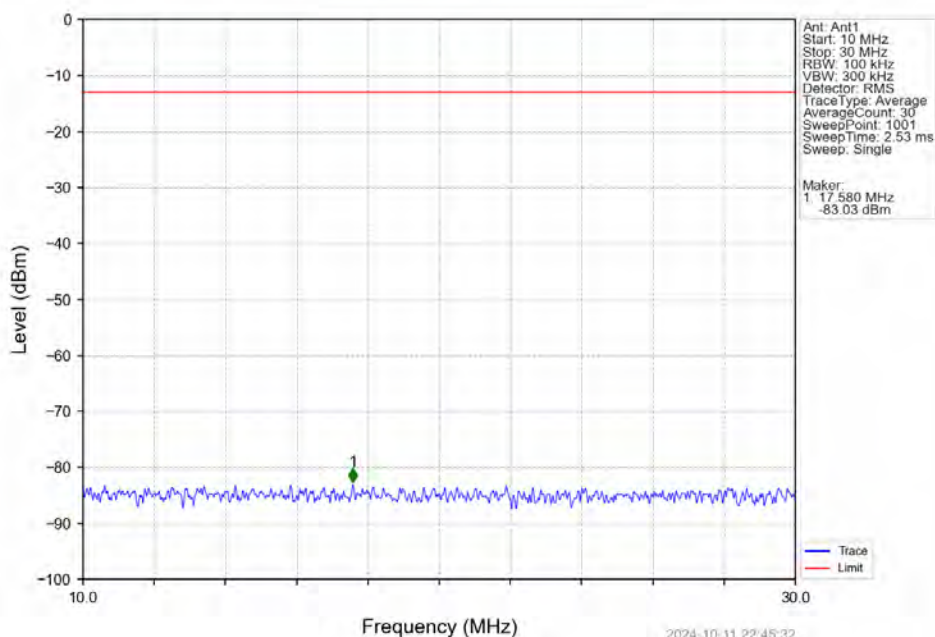
Band2 15MHz QPSK LCH 1857.5MHz RB 1 0 NTN
