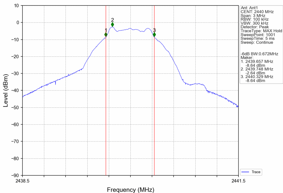
1M MCH 2440MHz Ant1 NTV
