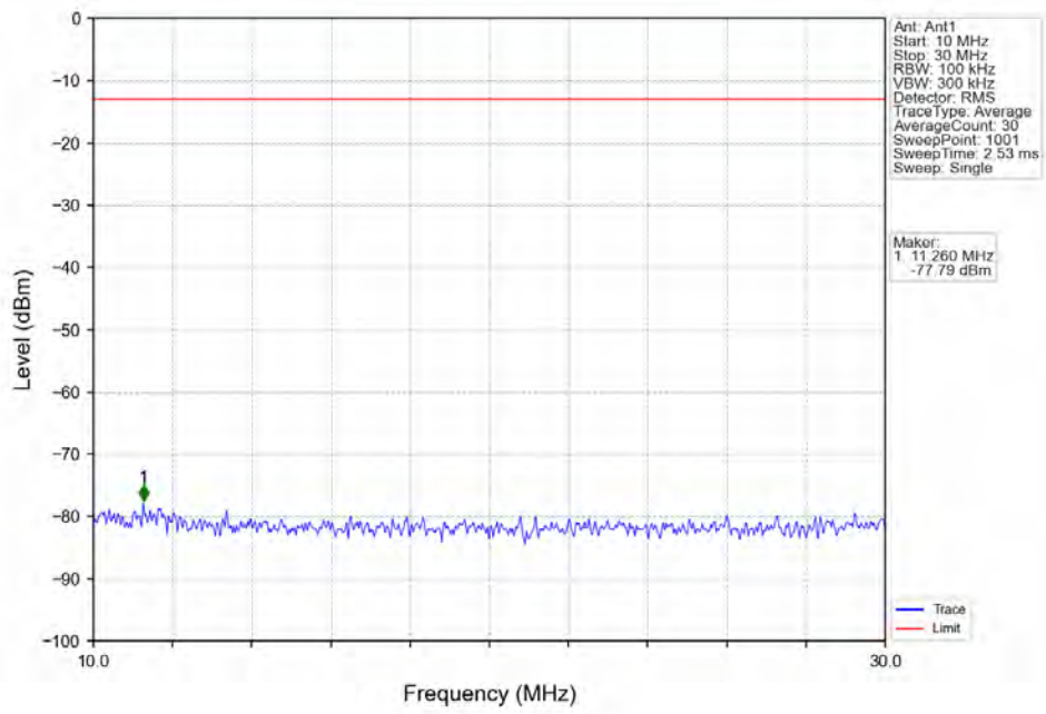
Band2_10MHz_16QAM_MCH_1880MHz_RB_1_0_NTNV
