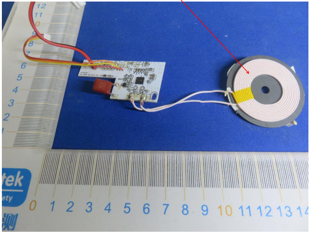
WPT ANT
