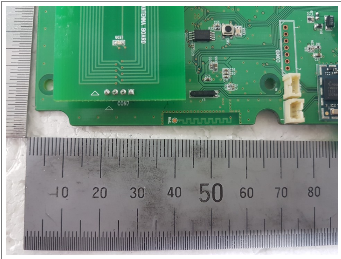
<BLE Antenna>
