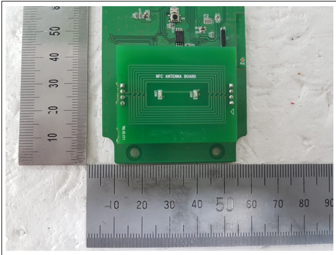
<NFC Antenna>
