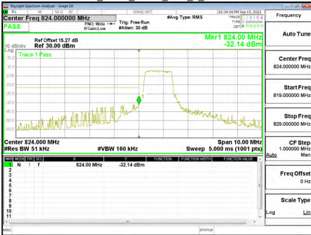
Band5_5MHz_QPSK_RB6_0_CH20425
