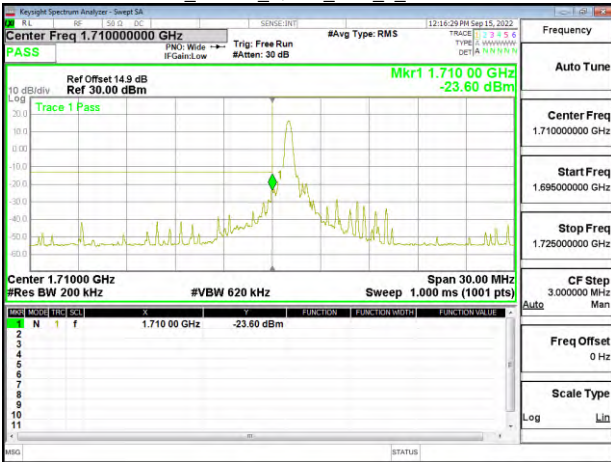
Band4_15MHz_QPSK_RB1_5_CH20325
