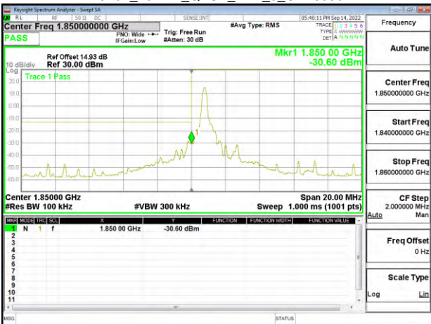
Band2_10MHz_QPSK_RB1_0_CH18650
