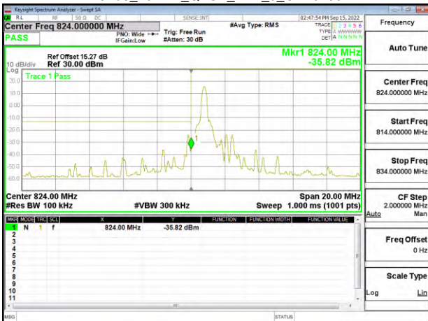
Band5_10MHz_QPSK_RB1_0_CH20450
