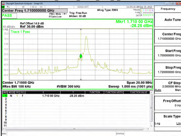
Band4_10MHz_QPSK_RB1_0_CH20000
