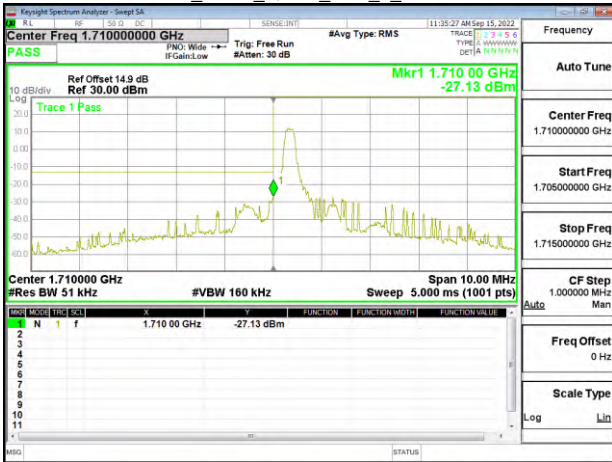
Band4_5MHz_QPSK_RB1_5_CH20375
