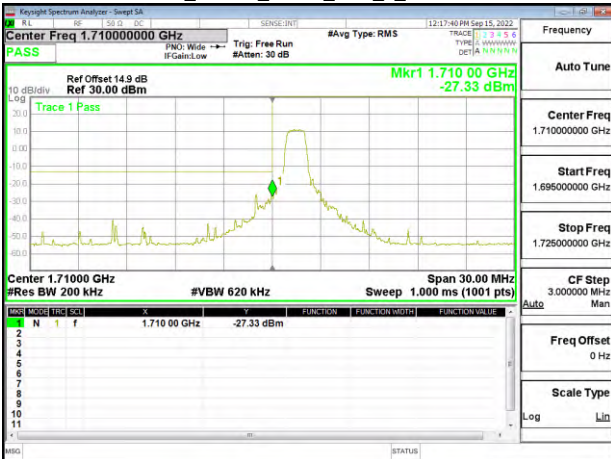
Band4_15MHz_QPSK_RB6_0_CH20025
