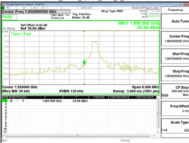
Band2_3MHz_QPSK_RB1_0_CH18615
