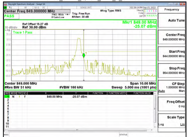
Band5_5MHz_QPSK_RB1_5_CH20625
