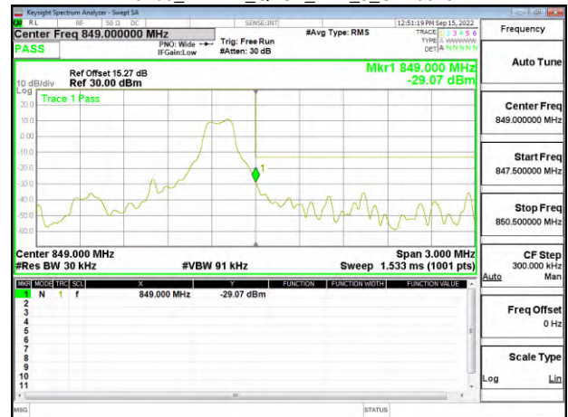
Band5_1.4MHz_QPSK_RB1_5_CH20643
