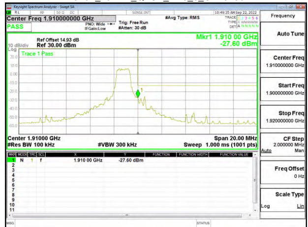
Band2_10MHz_QPSK_RB6_0_CH19150
