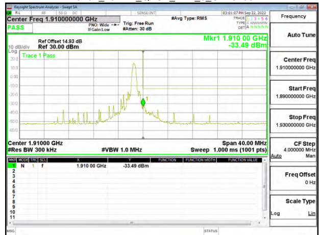
Band2_20MHz_QPSK_RB1_5_CH19100
