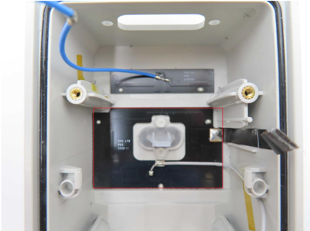
WWAN Antenna
