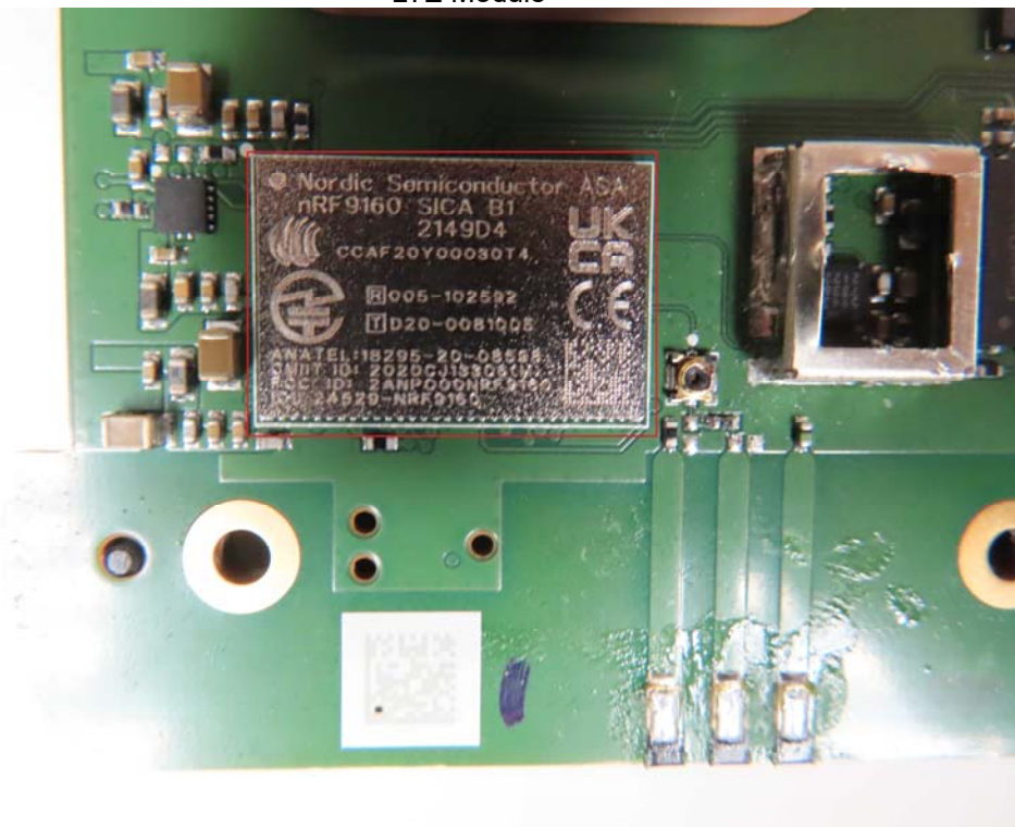
LTE Module
