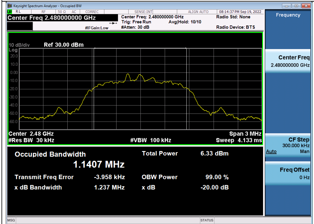
Test_Graph_EDR_ANT1_2480_3Mbps_OBW
