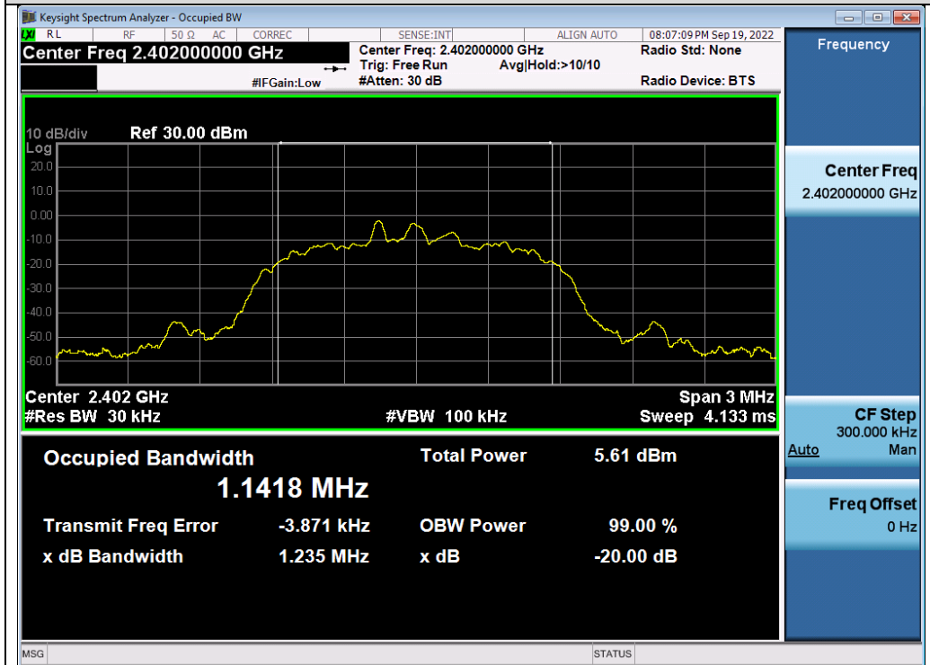
Test_Graph_EDR_ANT1_2402_3Mbps_OBW
