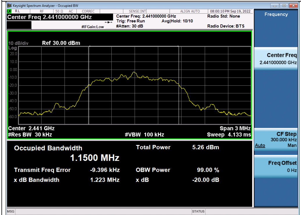
Test_Graph_EDR_ANT1_2441_2Mbps_OBW
