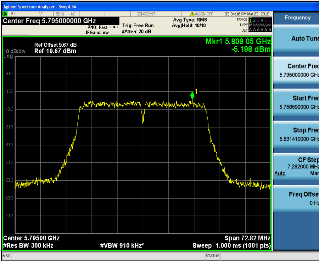
High 802.11ac(HT40)
