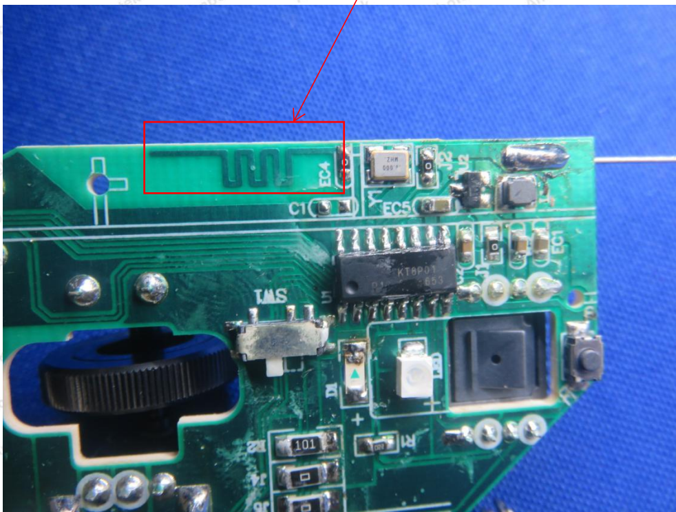
TX ANT
