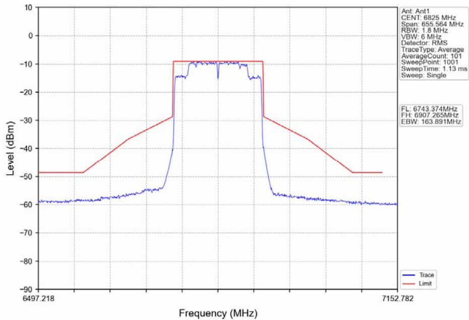
802.11ax(HEW160)_HCH_6825MHz_2xRU996_Left_Ant1_NTNV
