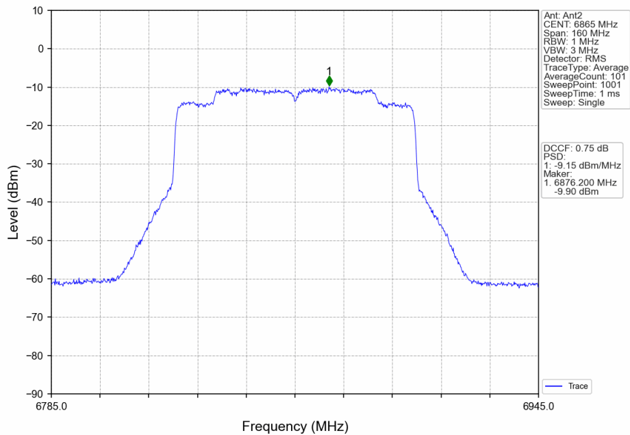
802.11ax(HEW80)_HCH_6865MHz_RU996_Left_Ant2_NTNV
