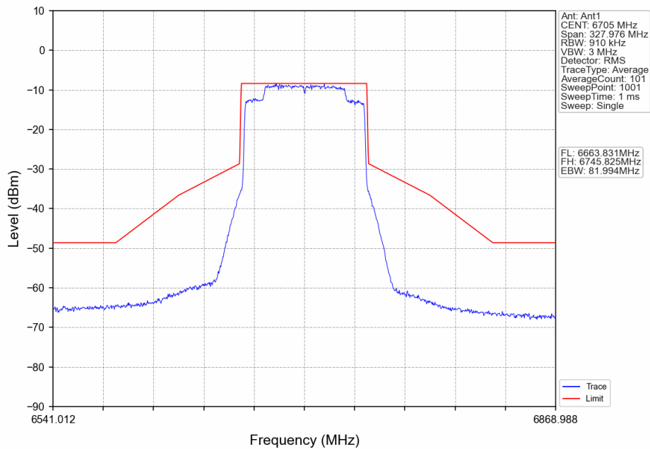
802.11ax(HEW80)_MCH_6705MHz_RU996_Left_Ant1_NTNV
