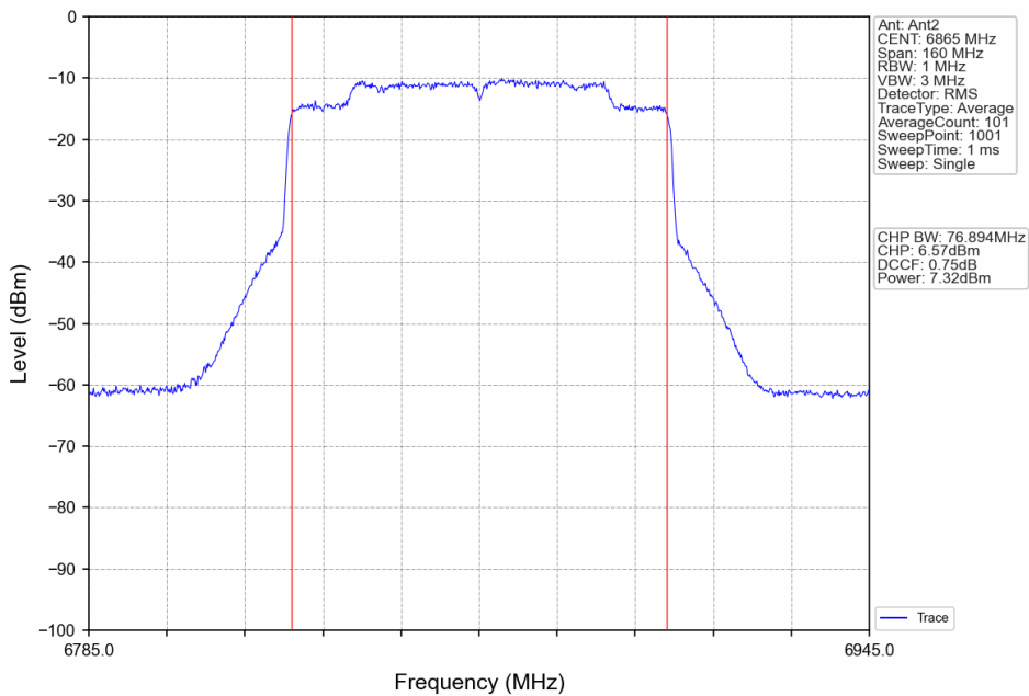
802.11ax(HEW80)_HCH_6865MHz_RU996_Left_Ant2_NTNV
