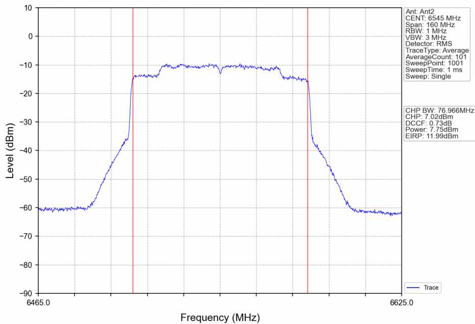
802.11ax(HEW80)_HCH_6545MHz_RU996_Left_Ant2_NTNV
