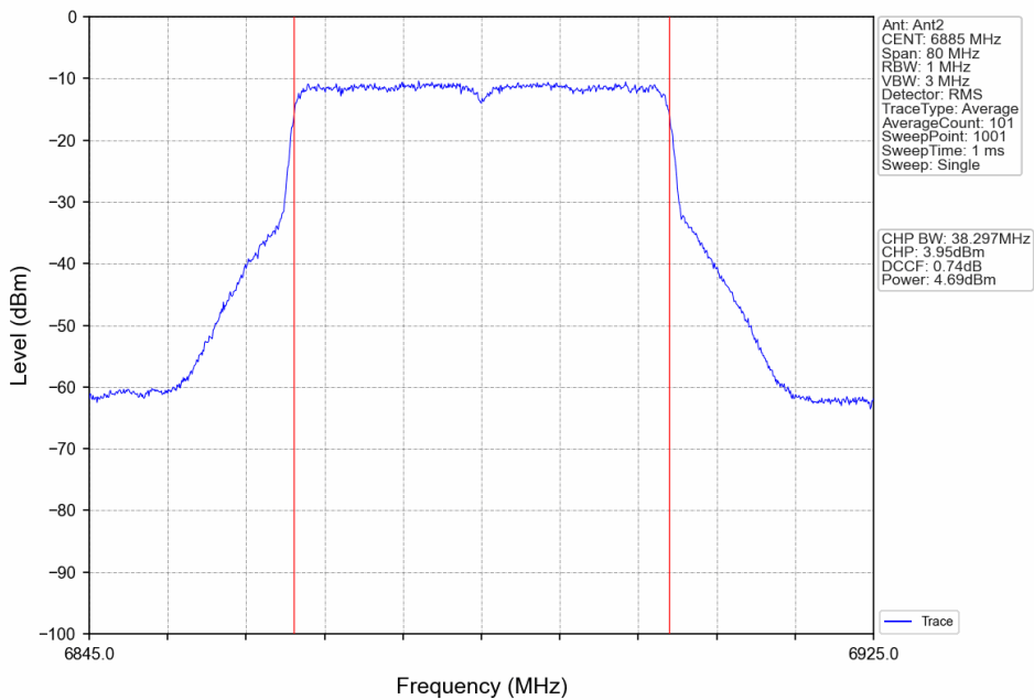
802.11ax(HEW40)_HCH_6885MHz_RU484_Left_Ant2_NTNV
