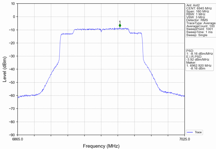
802.11ax(HEW80)_LCH_6945MHz_RU996_Left_Ant2_NTNV
