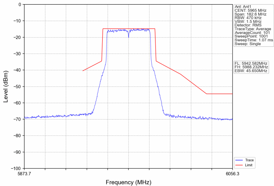
802.11ax(HEW40)_LCH_5965MHz_RU484_Left_Ant1_NTNV
