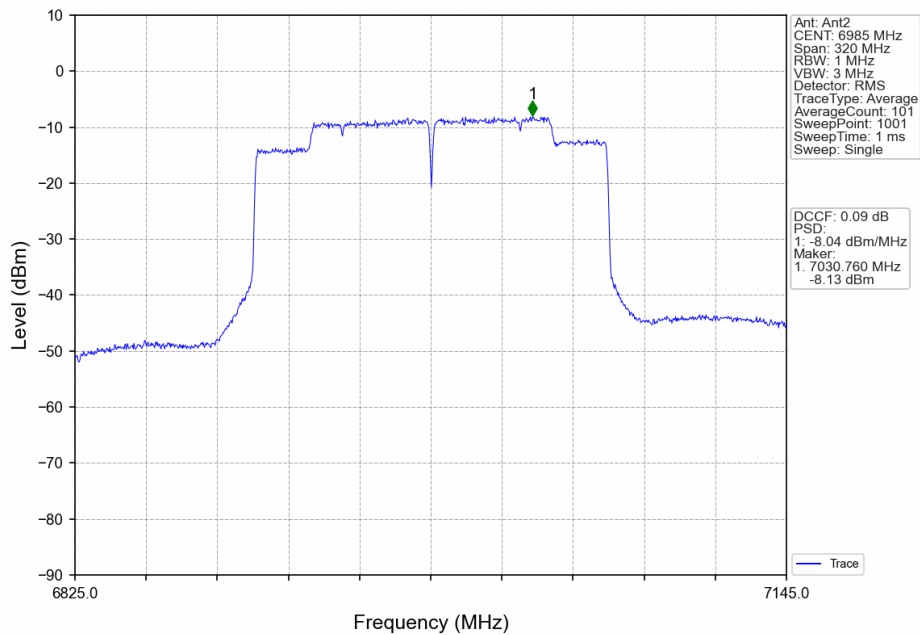
802.11ax(HEW160)_MCH_6985MHz_2xRU996_Left_Ant2_NTNV
