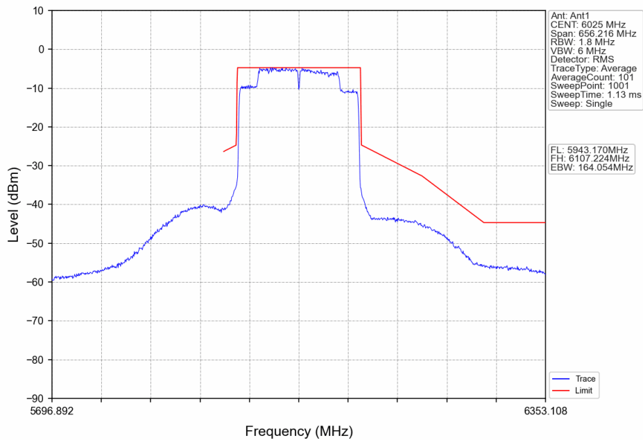
802.11ax(HEW160)_LCH_6025MHz_2xRU996_Left_Ant1_NTNV
