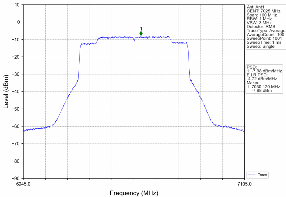
802.11ax(HEW80)_HCH_7025MHz_RU996_Left_Ant1_NTNV
