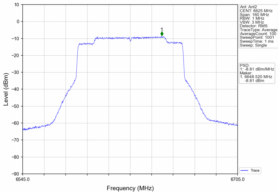
802.11ax(HEW80)_LCH_6625MHz_RU996_Left_Ant2_NTNV
