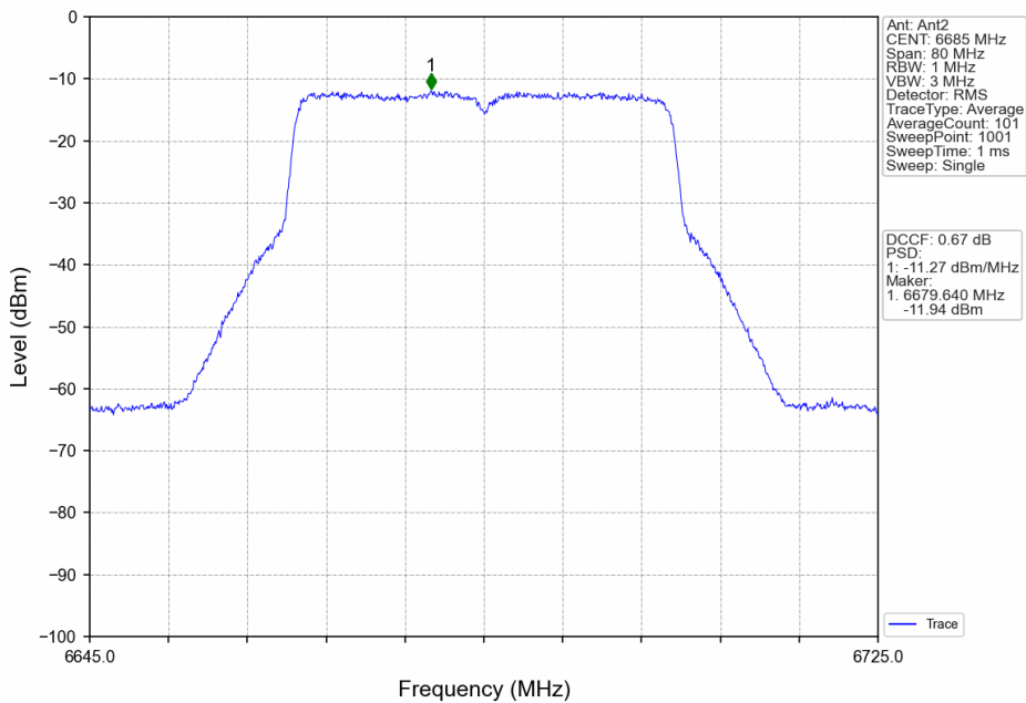
802.11ax(HEW40)_MCH_6685MHz_RU484_Left_Ant2_NTNV
