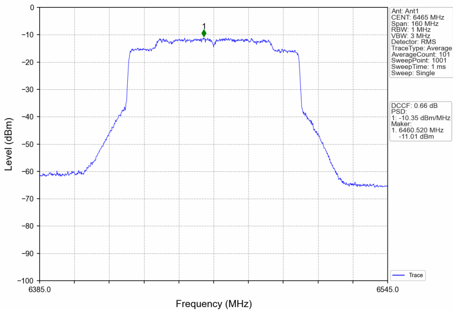
802.11ax(HEW80)_LCH_6465MHz_RU996_Left_Ant1_NTNV
