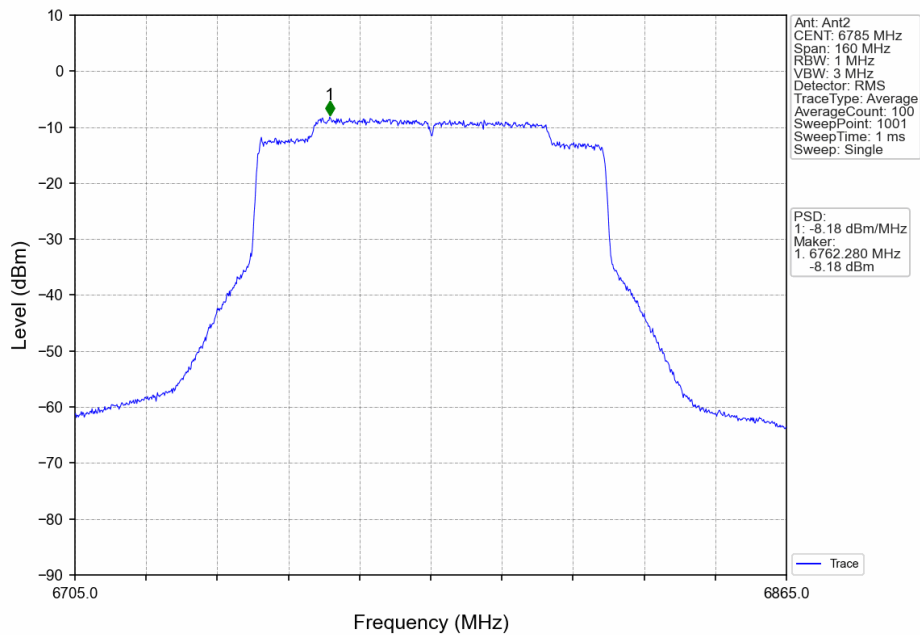
802.11ax(HEW80)_HCH_6785MHz_RU996_Left_Ant2_NTNV
