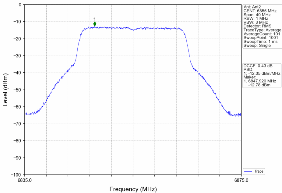
802.11ax(HEW20)_HCH_6855MHz_RU242_Left_Ant2_NTNV
