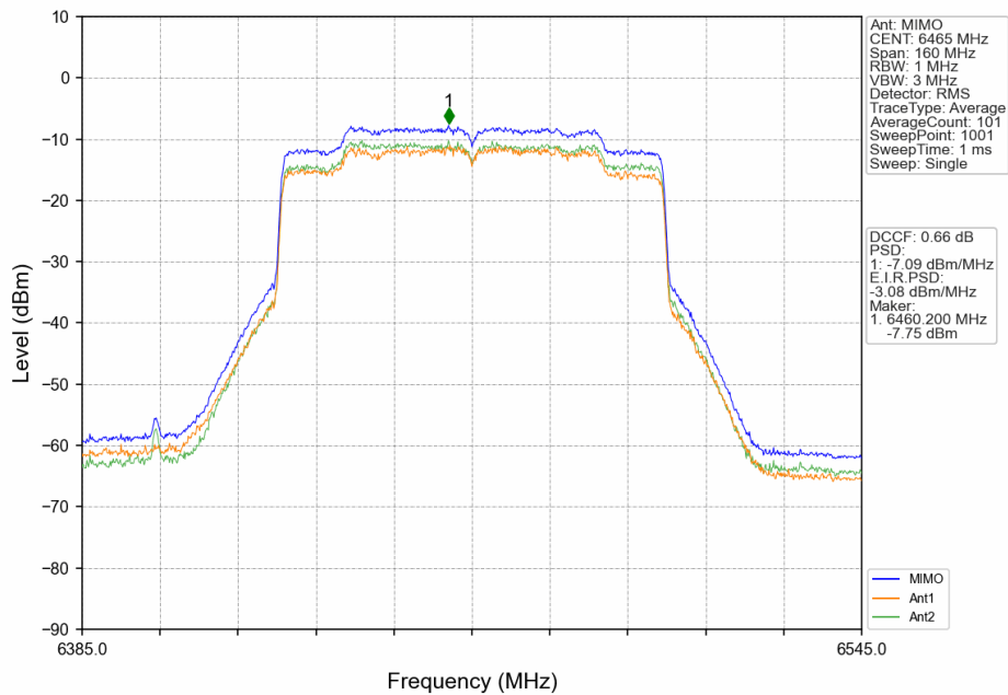
802.11ax(HEW80)_LCH_6465MHz_RU996_Left_MIMO_NTNV
