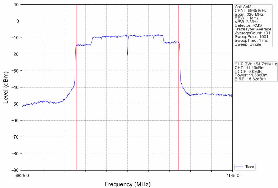
802.11ax(HEW160)_MCH_6985MHz_2xRU996_Left_Ant2_NTNV
