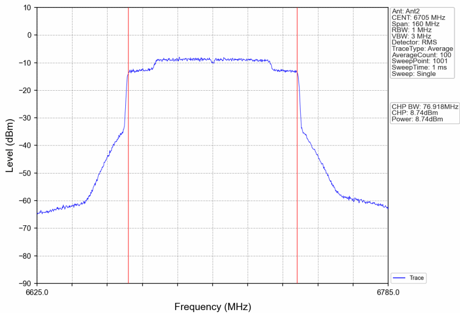
802.11ax(HEW80)_MCH_6705MHz_RU996_Left_Ant2_NTNV
