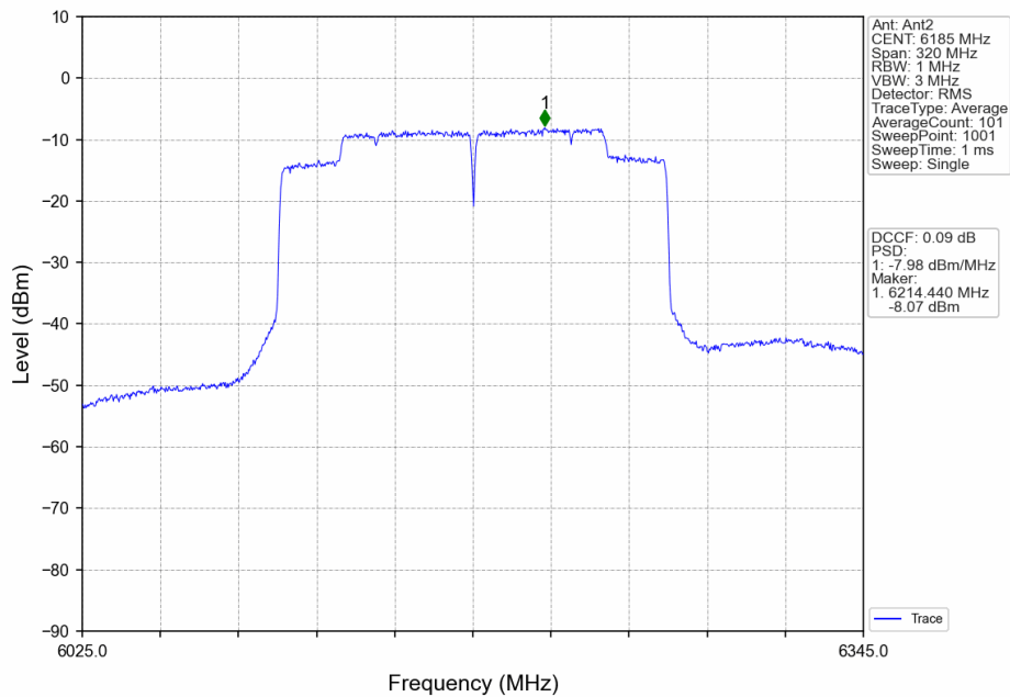
802.11ax(HEW160)_MCH_6185MHz_2xRU996_Left_Ant2_NTNV
