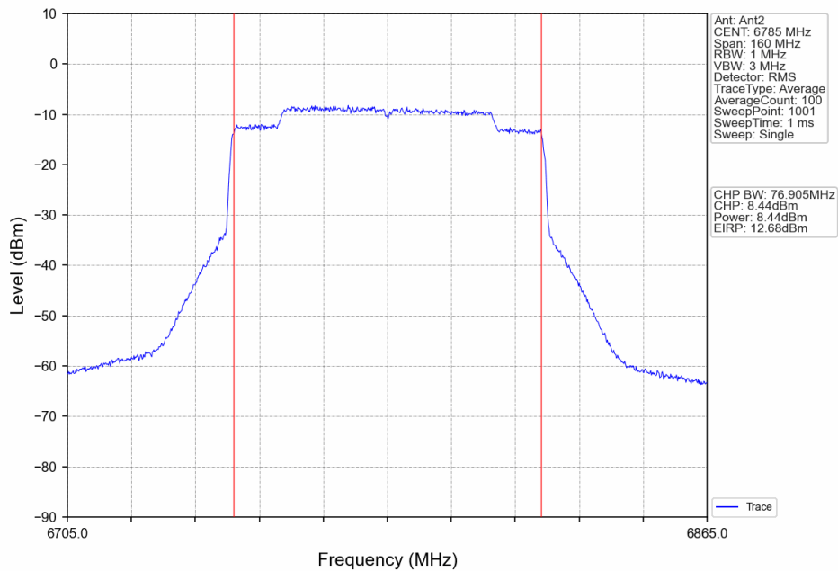
802.11ax(HEW80)_HCH_6785MHz_RU996_Left_Ant2_NTNV
