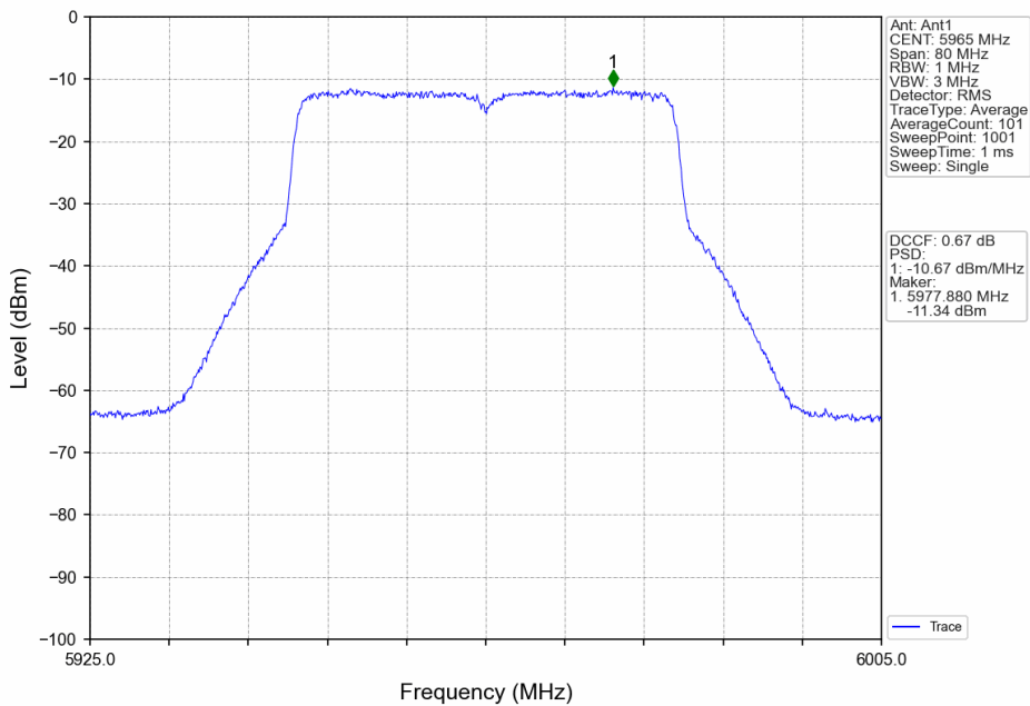
802.11ax(HEW40)_LCH_5965MHz_RU484_Left_Ant1_NTNV
