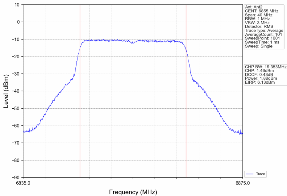
802.11ax(HEW20)_HCH_6855MHz_RU242_Left_Ant2_NTNV
