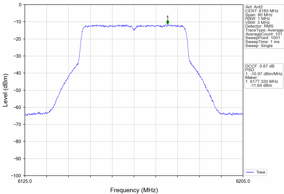
802.11ax(HEW40)_MCH_6165MHz_RU484_Left_Ant2_NTNV
