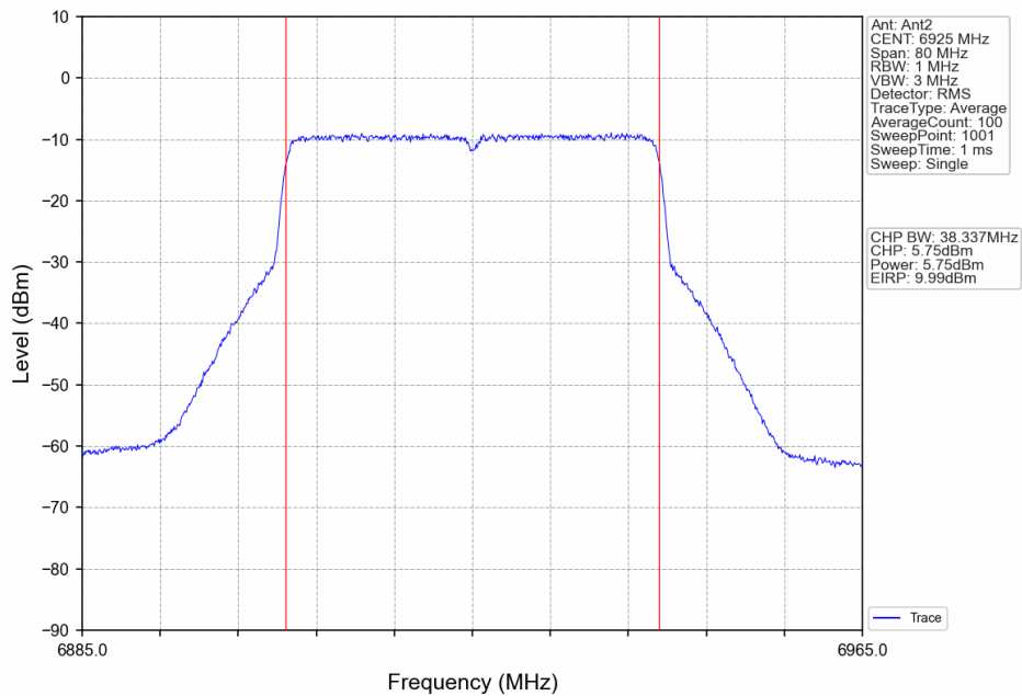
802.11ax(HEW40)_LCH_6925MHz_RU484_Left_Ant2_NTNV
