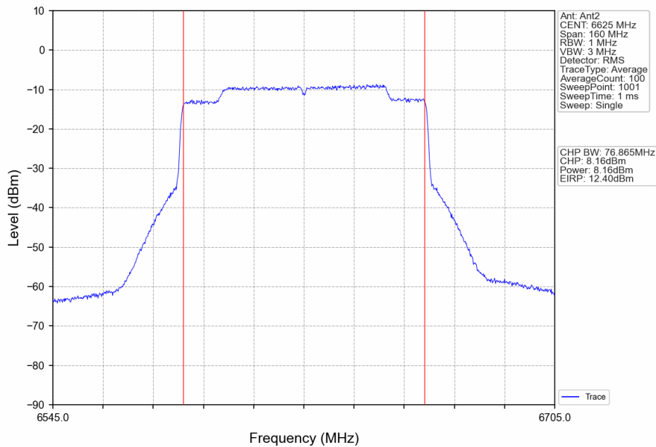
802.11ax(HEW80)_LCH_6625MHz_RU996_Left_Ant2_NTNV
