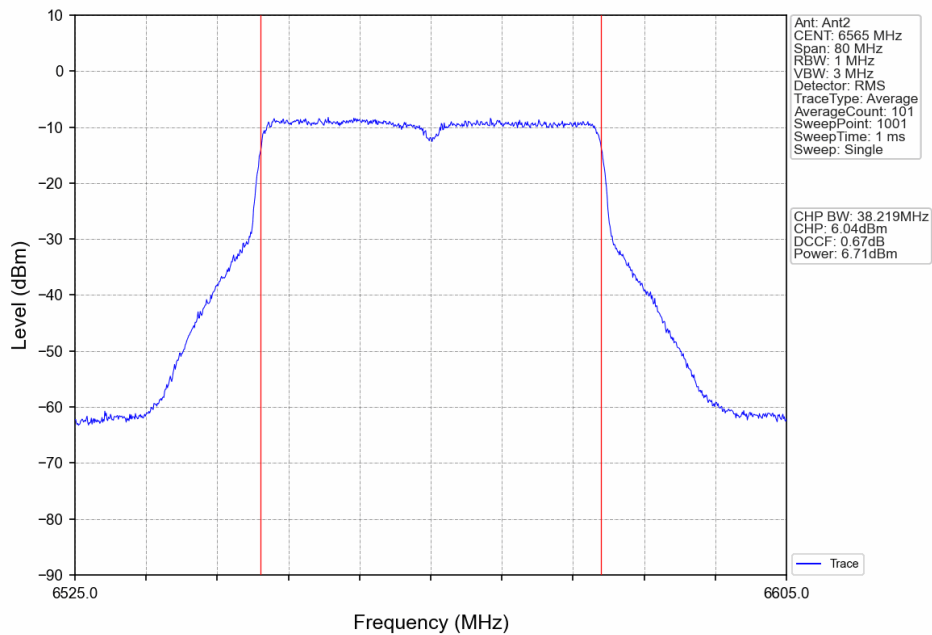
802.11ax(HEW40)_LCH_6565MHz_RU484_Left_Ant2_NTNV
