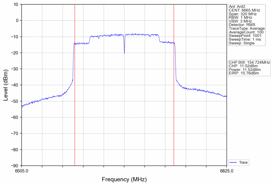
802.11ax(HEW160)_MCH_6665MHz_2xRU996_Left_Ant2_NTNV
