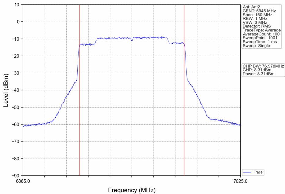
802.11ax(HEW80)_LCH_6945MHz_RU996_Left_Ant2_NTNV
