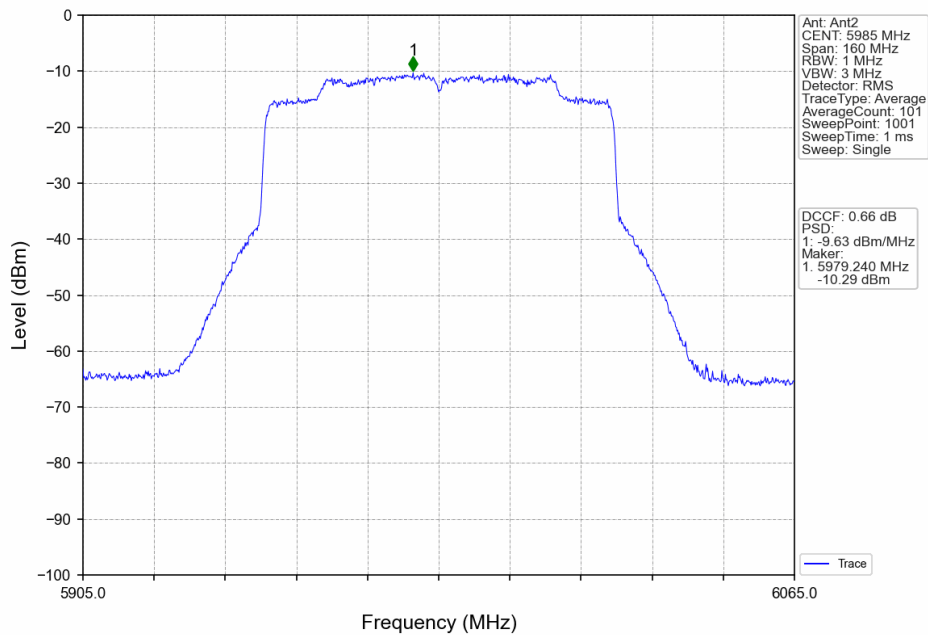
802.11ax(HEW80)_LCH_5985MHz_RU996_Left_Ant2_NTNV
