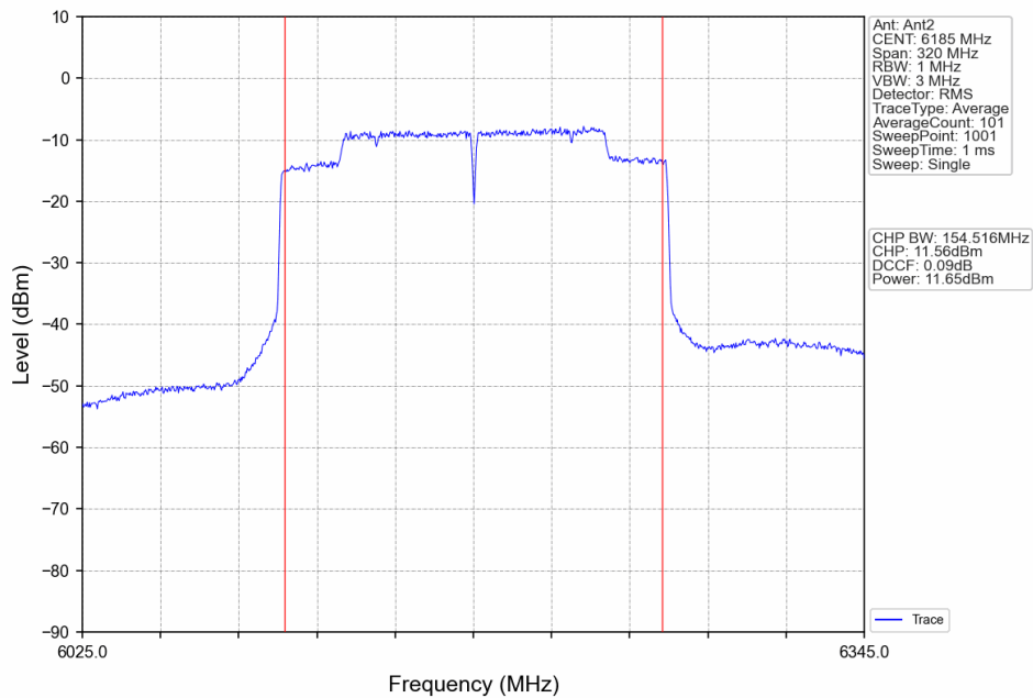
802.11ax(HEW160)_MCH_6185MHz_2xRU996_Left_Ant2_NTNV
