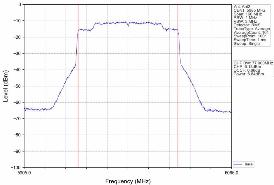
802.11ax(HEW80)_LCH_5985MHz_RU996_Left_Ant2_NTNV
