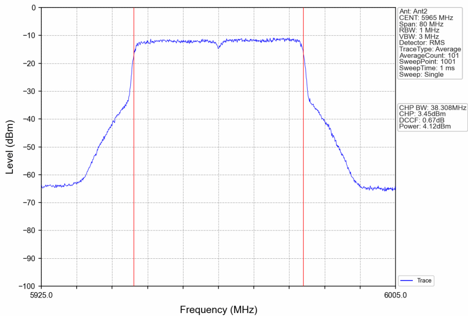
802.11ax(HEW40)_LCH_5965MHz_RU484_Left_Ant2_NTNV
