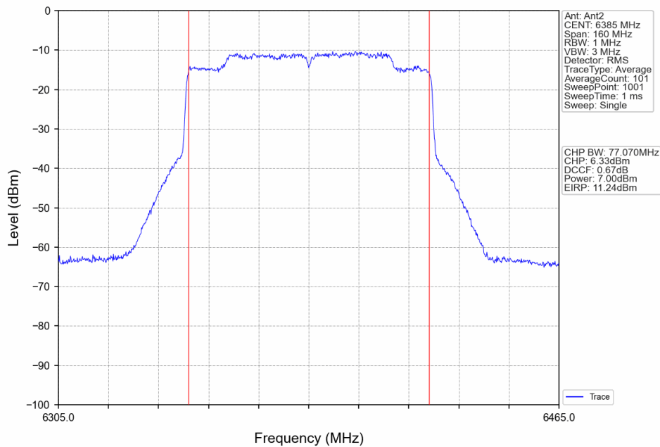
802.11ax(HEW80)_HCH_6385MHz_RU996_Left_Ant2_NTNV
