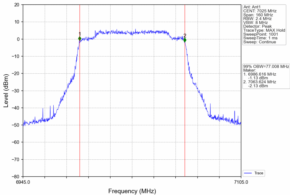
802.11ax(HEW80)_HCH_7025MHz_RU996_Left_Ant1_NTNV
