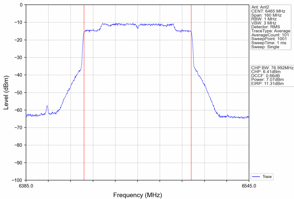
802.11ax(HEW80)_LCH_6465MHz_RU996_Left_Ant2_NTNV
