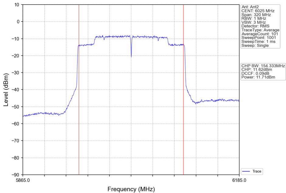
802.11ax(HEW160)_LCH_6025MHz_2xRU996_Left_Ant2_NTNV
