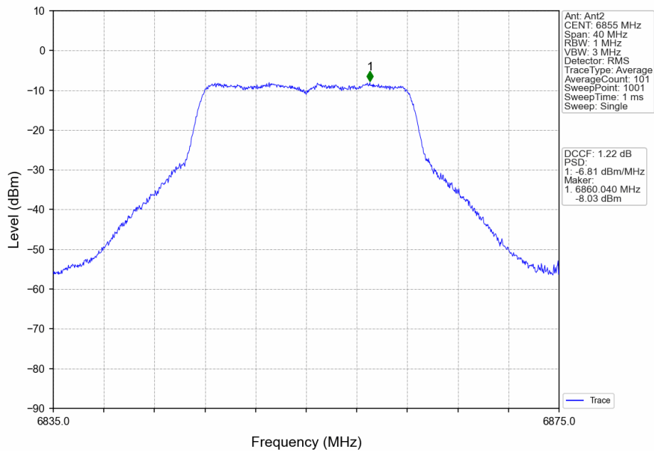
802.11ax(HEW20)_HCH_6855MHz_RU242_Left_Ant2_NTNV
