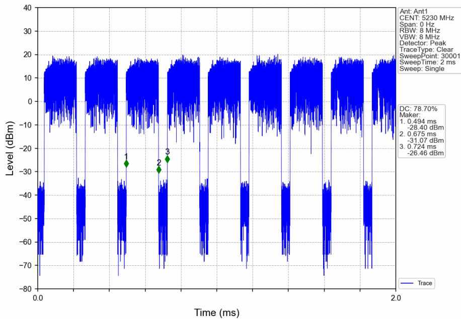
802.11ax(HEW40)_HCH_5230MHz_RU484_Left_Ant1_NTNV
