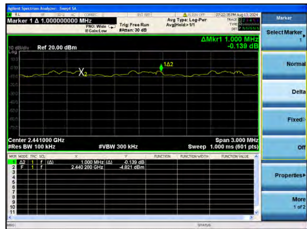
\pi/4 -DQPSK
