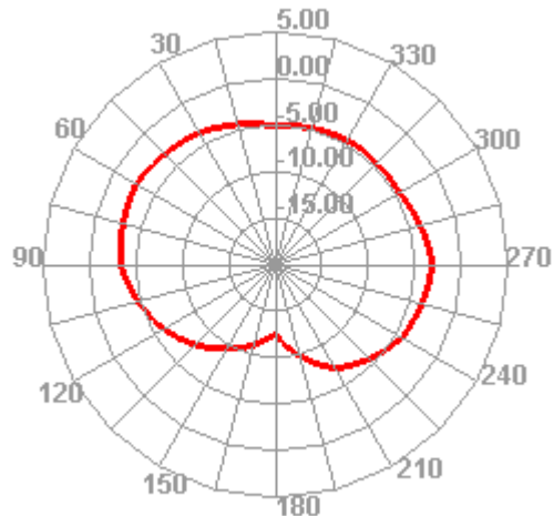
2440.000MHz E2
