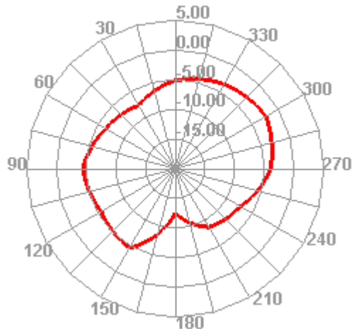
2440.000MHz E1
