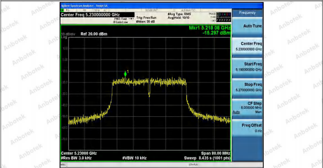
11N40SISO_Ant1_5230
