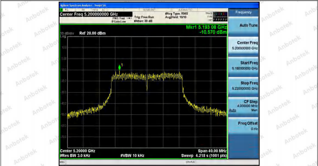
11N20SISO_Ant2_5200
