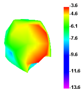
2480.000MHz
