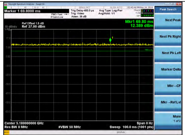
802.11n HT20
