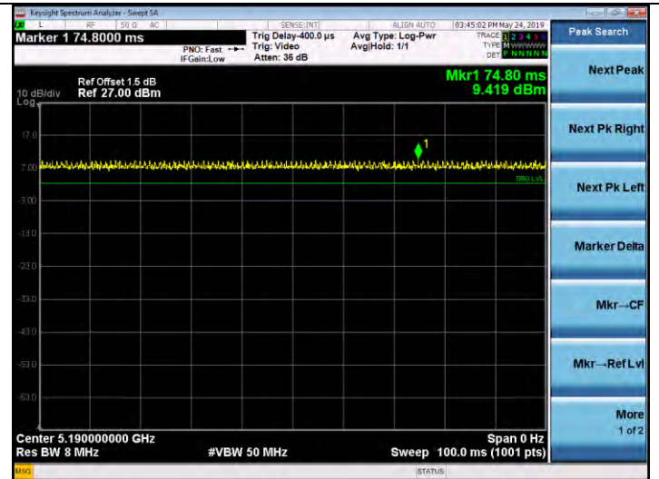
802.11n HT40
