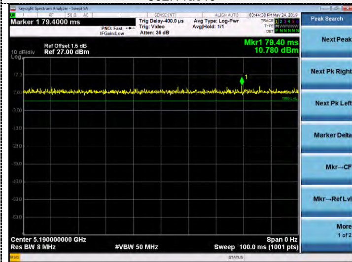
802.11ac40
