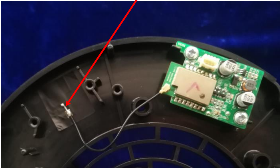
Antenna
