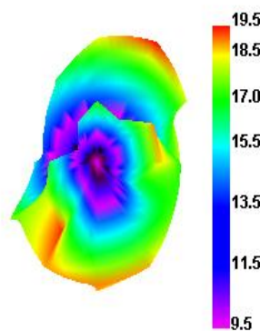
LTE2 19150 TRP
