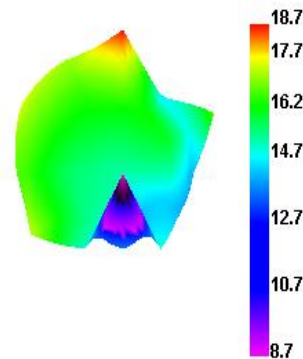
LTE7 21400 TRP
