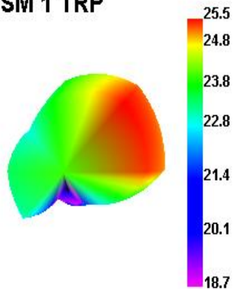
EGSM 1 TRP
