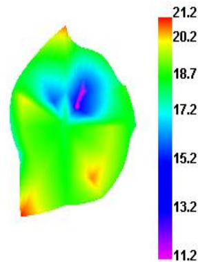
LTE3 19900 TRP
