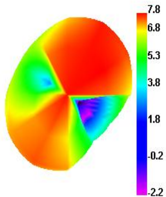
LTE12 23060 TRP
