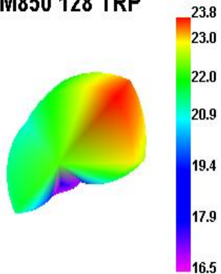
GSM850 128 TRP
