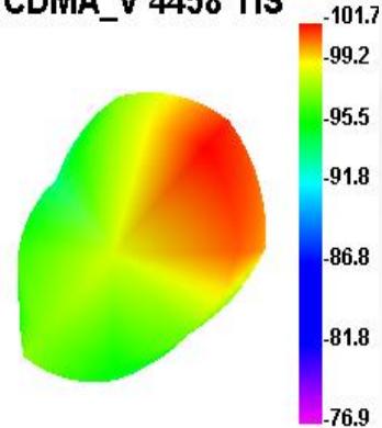
WCDMA_V 4458 TIS
