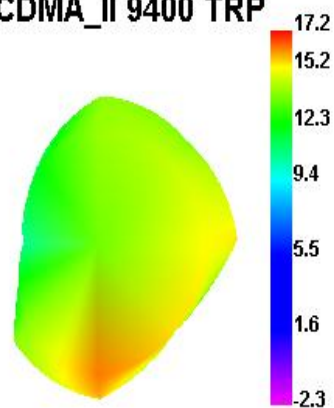
WCDMA_II 9400 TRP
