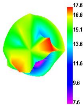
LTE3 19250 TRP
