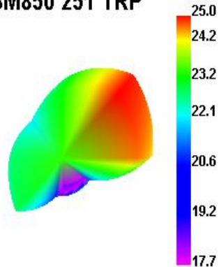
GSM850 251 TRP
