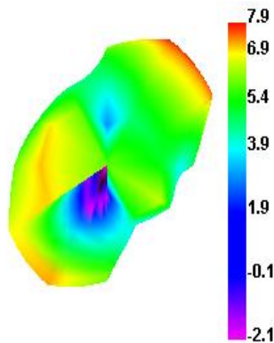
LTE12 23095 TRP
