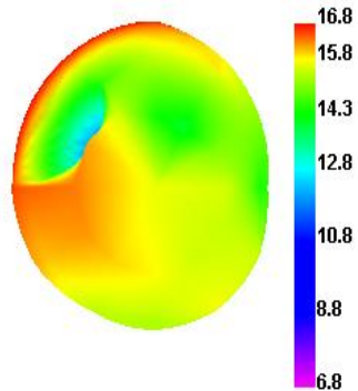
LTE7 21100 TRP
