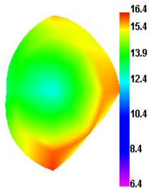
WCDMA_I 9612 TRP
