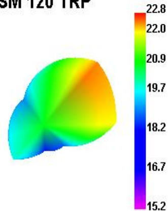
EGSM 120 TRP
