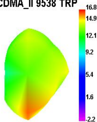
WCDMA_II 9538 TRP
