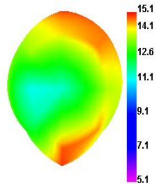
WCDMA_I 9888 TRP
