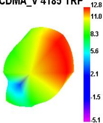
WCDMA_V 4185 TRP
