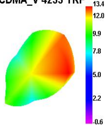
WCDMA_V 4233 TRP
