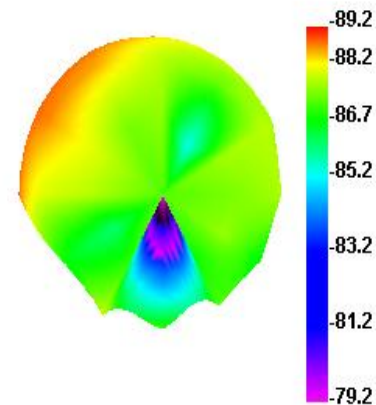
LTE7 3400 TIS
