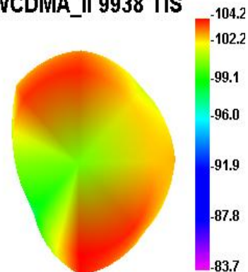
WCDMA_II 9938 TIS
