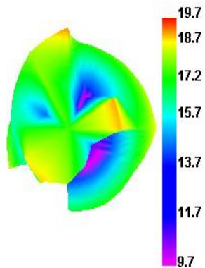
LTE4 20000 TRP
