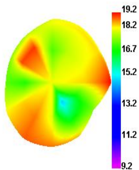
LTE2 18650 TRP
