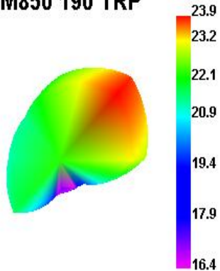
GSM850 190 TRP
