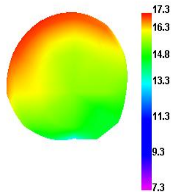
LTE7 20800 TRP
