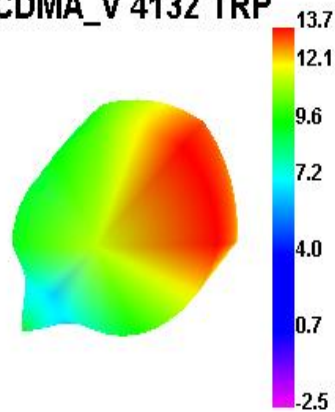
WCDMA_V 4132 TRP
