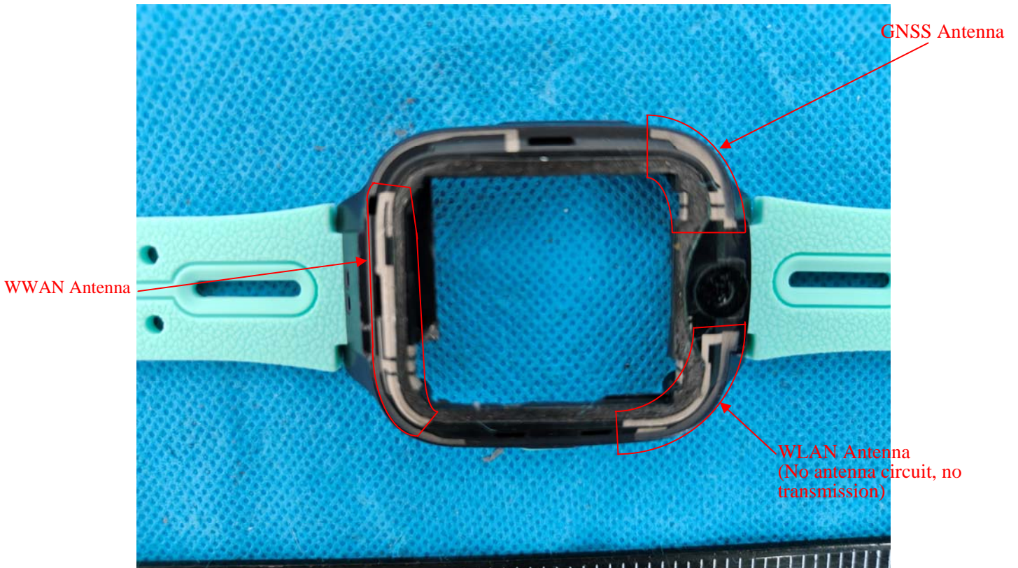
Antenna
