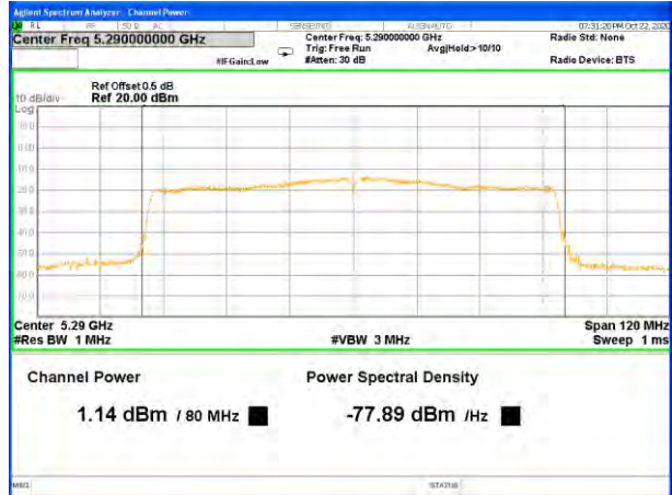
5290MHz_Ant B
