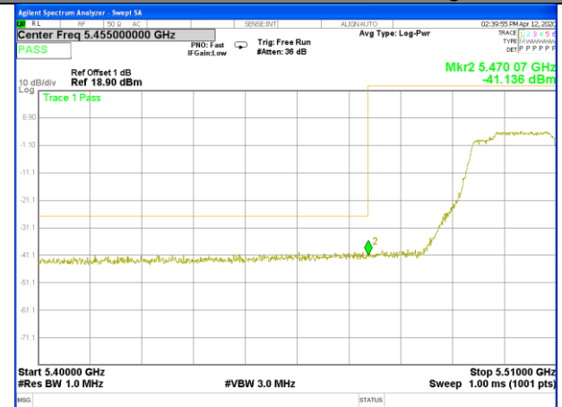
W56_11ac40_Lower_Band edge
