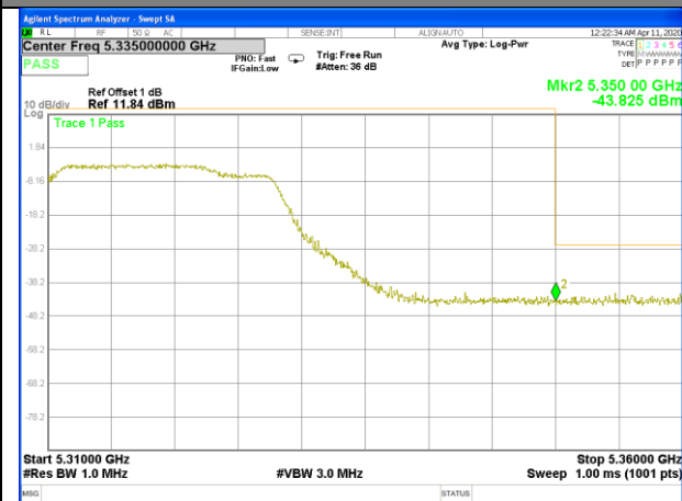
W53_11ac40_Higher_Band edge
