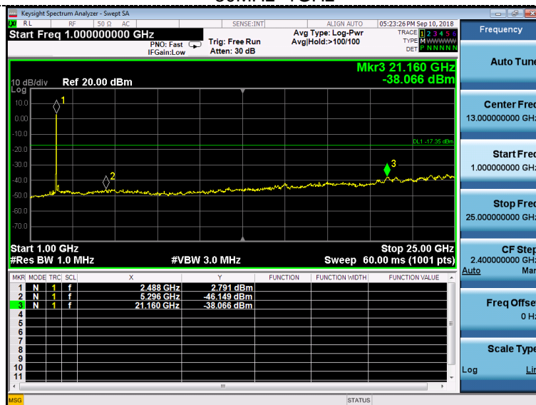
1GHz~25GHz
