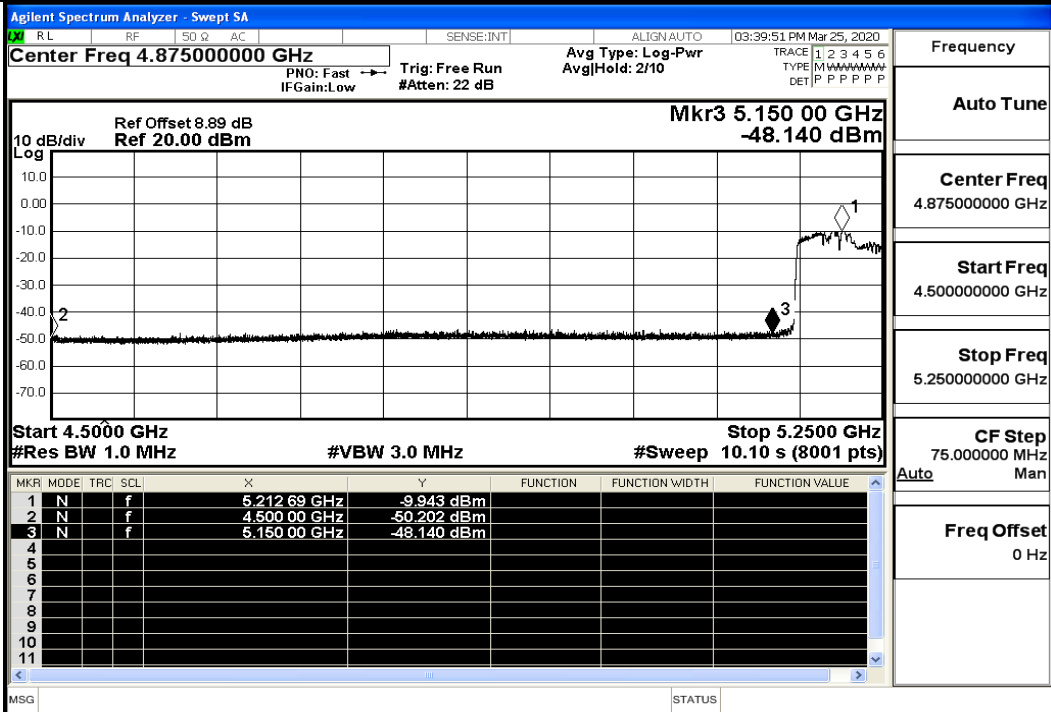
IEEE 802.11ac80 / Channel 42 / 5210MHz / Peak
