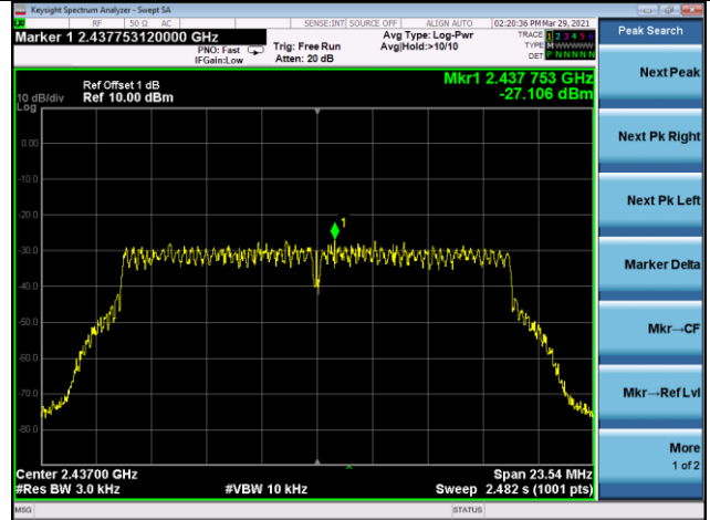
IEEE 802.11n(HT20) - 2437MHz
