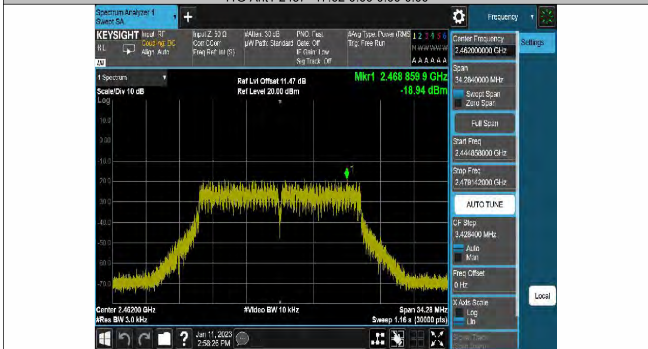
11G-Ant1-2462--18.94-0.00-0.00-0.00
