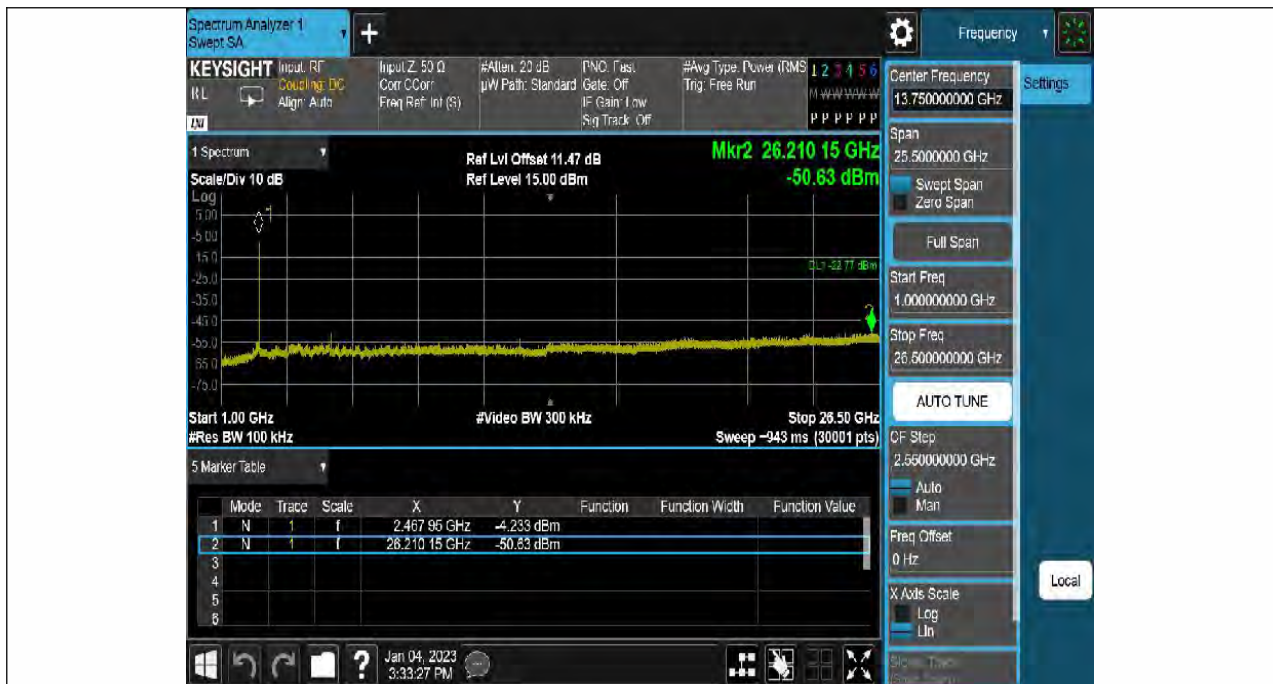
11N20SISO-Ant1-2462-1000~26500~-2.77
