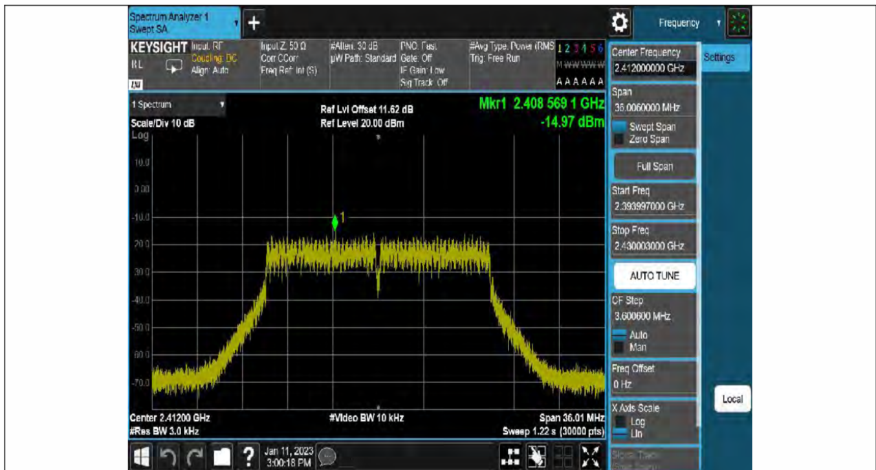
11N20SISO-Ant1-2412--14.97-0.00-0.00-0.00
