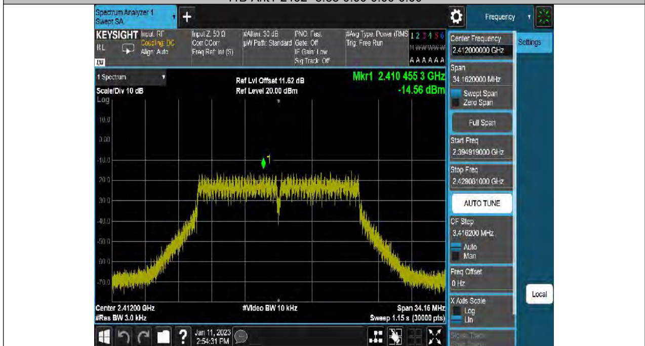
11G-Ant1-2412--14.56-0.00-0.00-0.00
