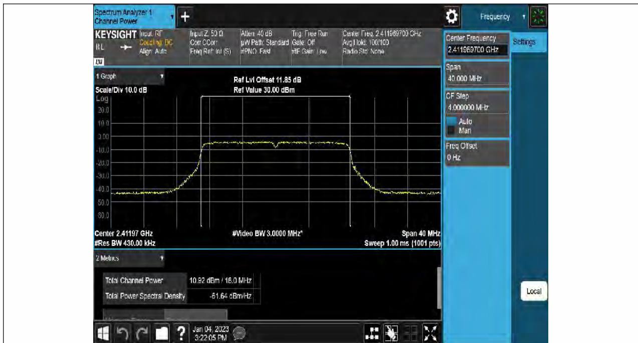
11N20SISO-Ant1-2412-----10.69-94.80-0.23
