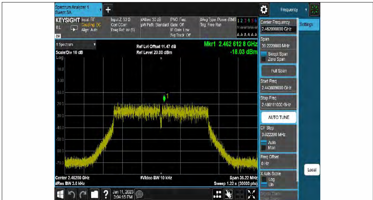
11N20SISO-Ant1-2462--18.03-0.00-0.00-0.00
