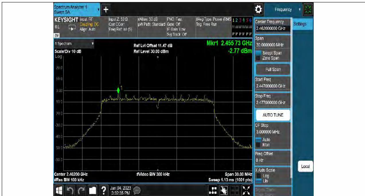
11N20SISO-Ant1-2462-0~Reference--2.77
