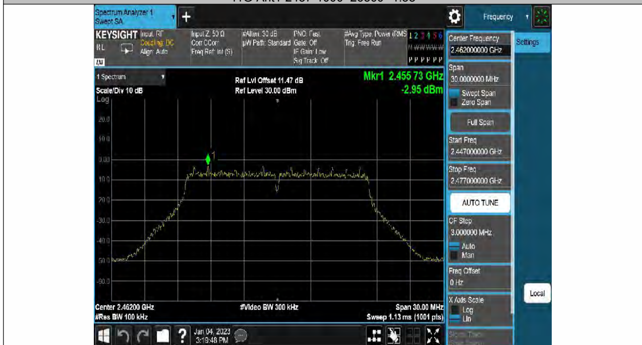
11G-Ant1-2462-0~Reference--2.95
