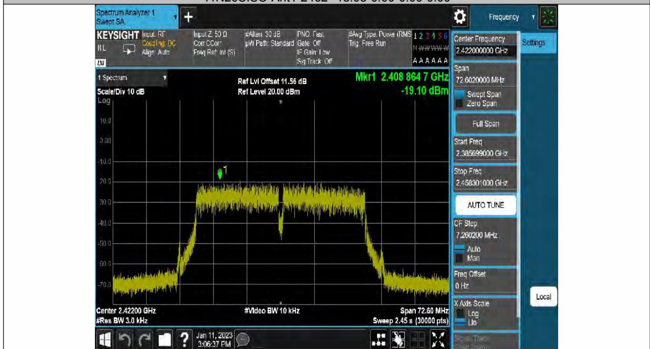
11N40SISO-Ant1-2422--19.10-0.00-0.00-0.00
