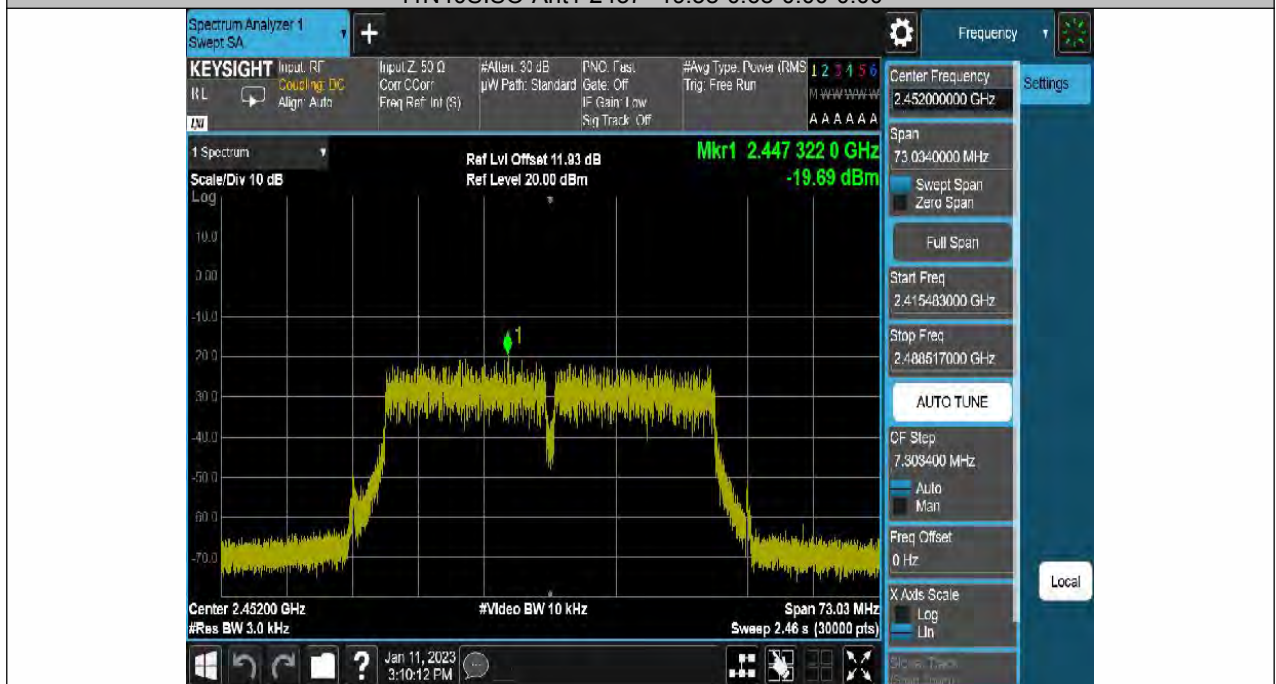
11N40SISO-Ant1-2452--20.15-0.46-0.00-0.00
