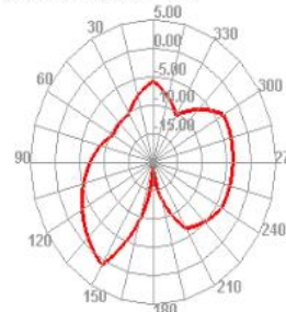
2450.000MHz E1
