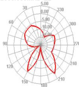
2500.000MHz E2
