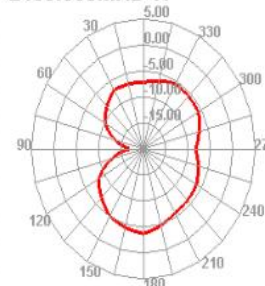
2450.000MHz E2
