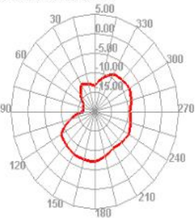
2400.000MHz E2
