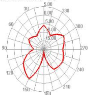
2400.000MHz E1
