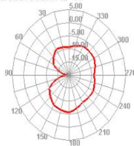
2425.000MHz H
