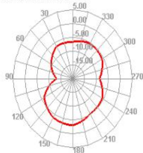
2475.000MHz E2
