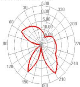
2425.000MHz E2
