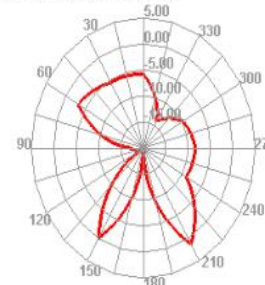
2450.000MHz E2
