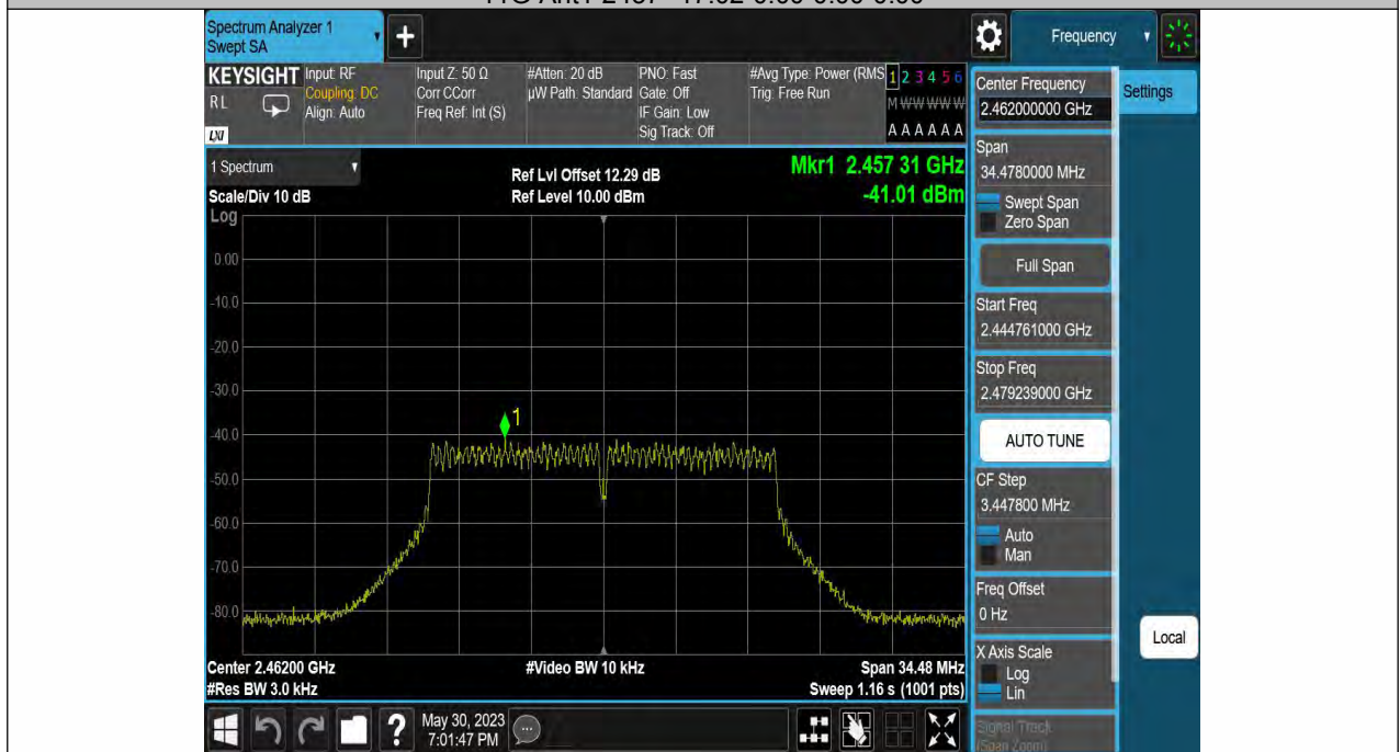
11G-Ant1-2462--18.94-0.00-0.00-0.00
