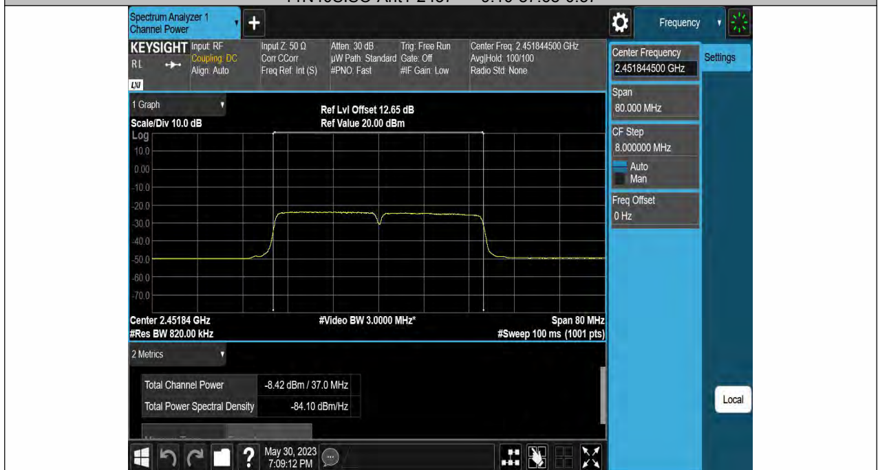
11N40SISO-Ant1-2452-----8.21-89.17-0.50
