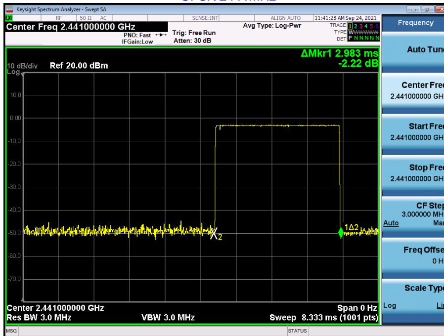
GFSK 2441MHz
