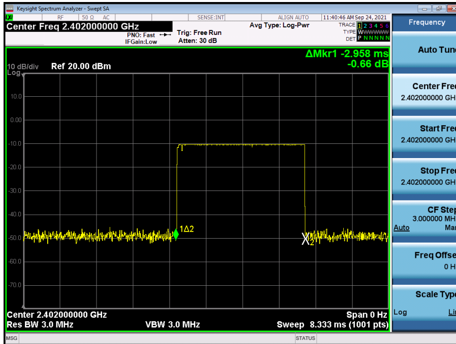
GFSK 2402MHz
