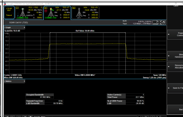
60MHz / 16QAM
