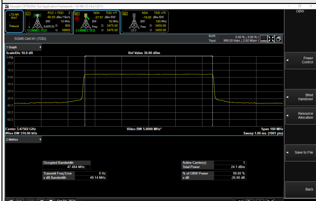
50MHz / 16QAM
