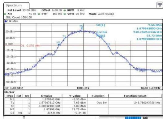
EDGE1900-661-0-PASS
