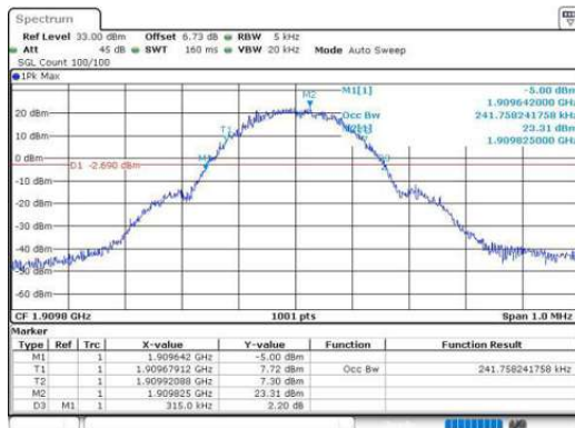
EDGE1900-810-0-PASS
