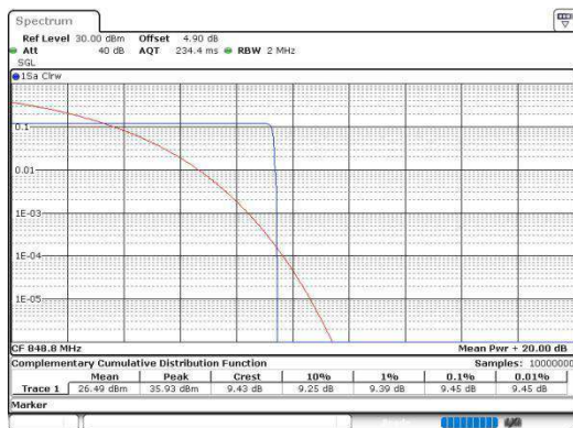
GSM850-251-5-PASS
