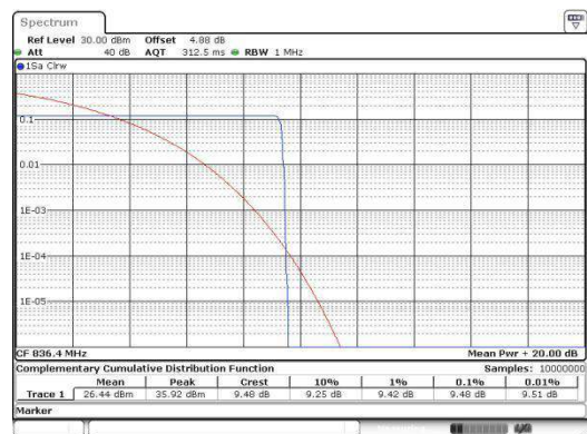
GSM850-189-5-PASS
