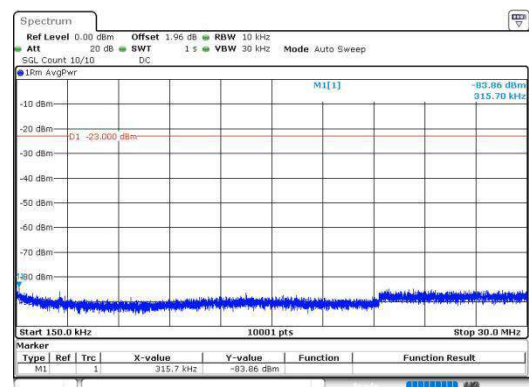
GSM850-189-5-0.15~30MHz-PASS
