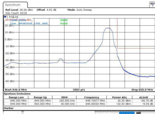
Band5_3MHz_16QAM_20635_15RB#0
