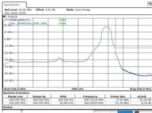
Band5_3MHz_QPSK_20635_15RB#0
