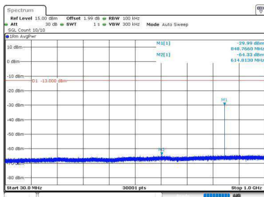
EDGE850-251-5-30~1000MHz-PASS
