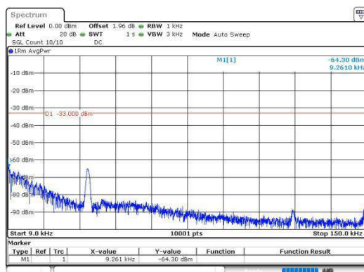
GSM850-189-5-0.009~0.15MHz-PASS
