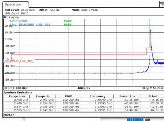
Band41_5MHz_QPSK_40065_25RB#0
