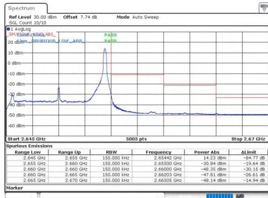
Band41_10MHz_QPSK_41190_50RB#0
