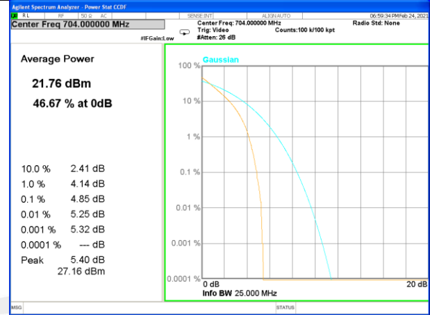
Band 12_50_Q16_Low
