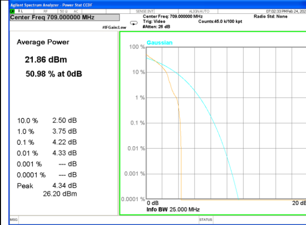
Band 17_1_Q16_Low
