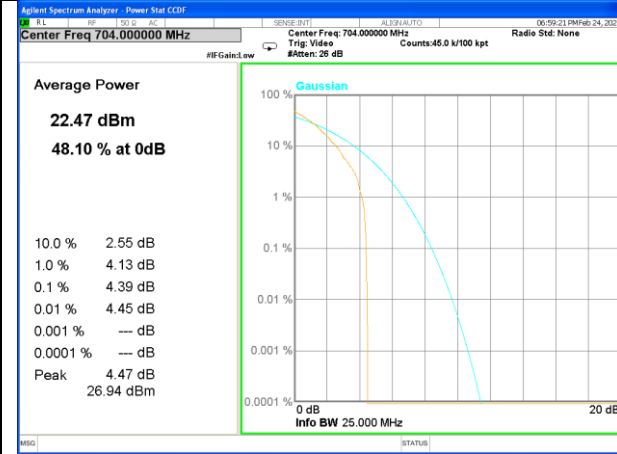
Band 12_1_Q16_Low
