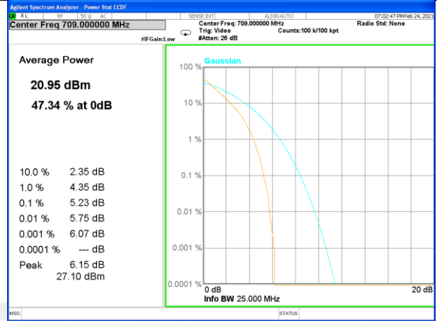
Band 17_50_Q16_Low
