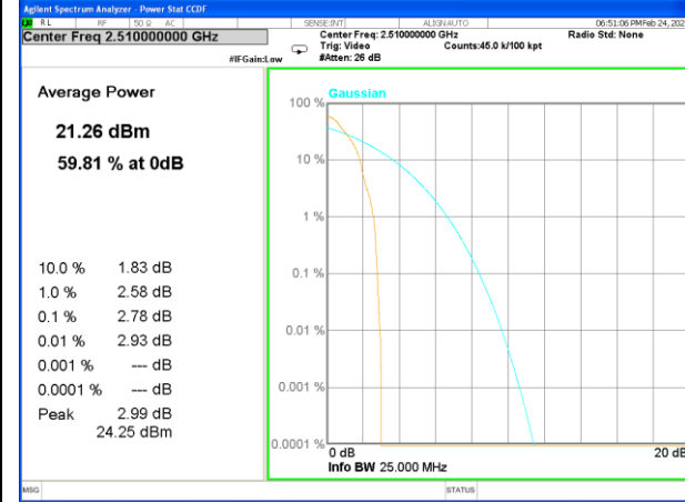
Band 7_1_Q16_Low
