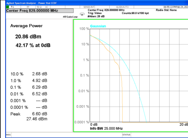
Band 5_1_Q16_Low
