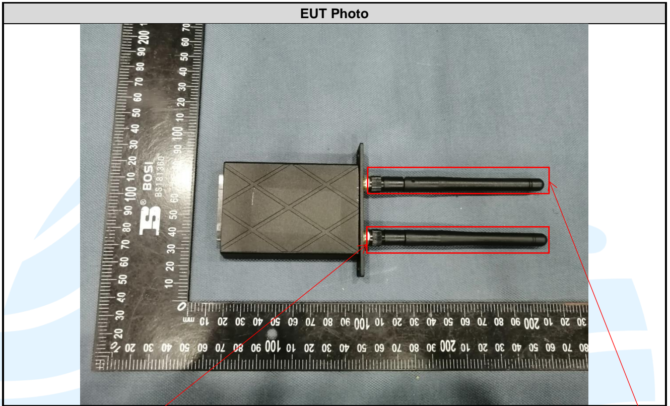
BT/WIFI Antenna 0
