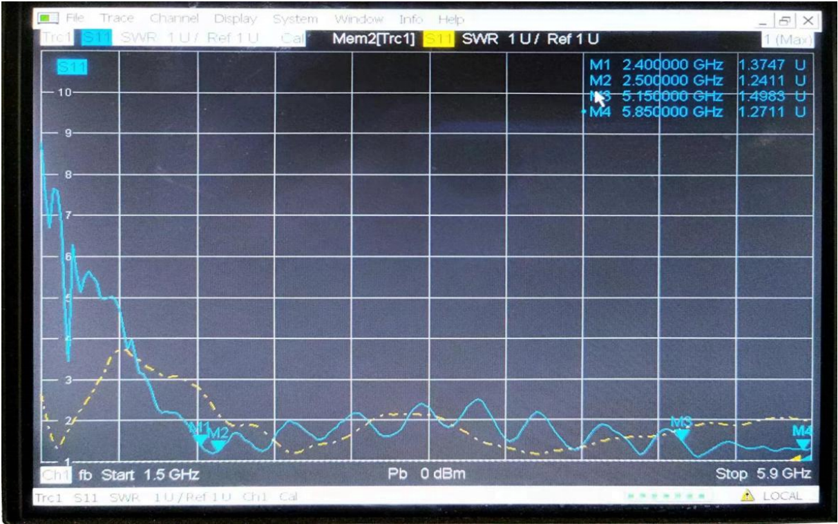
VSWR<2
